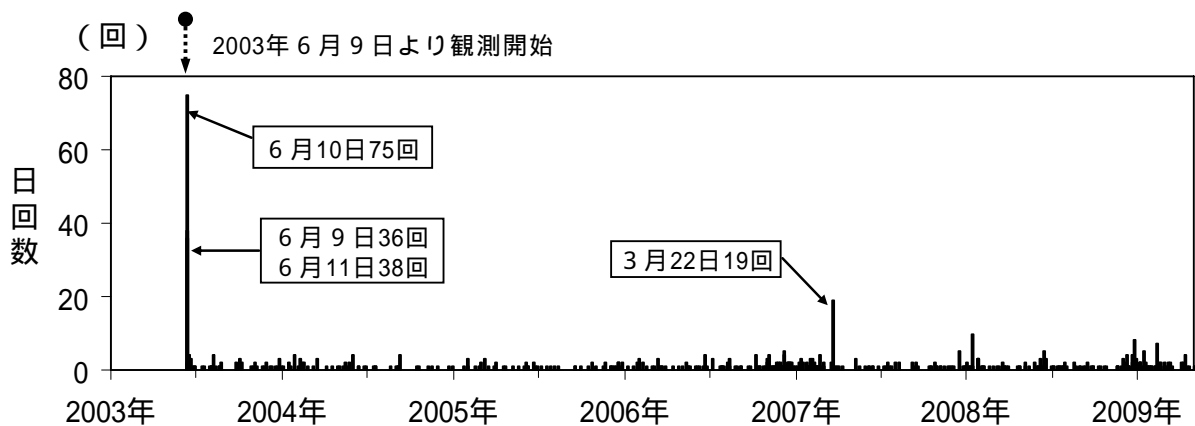
図 2 秋田駒ヶ岳 日別地震回数（2003 年 6 月 9 日～2009 年 4 月）
