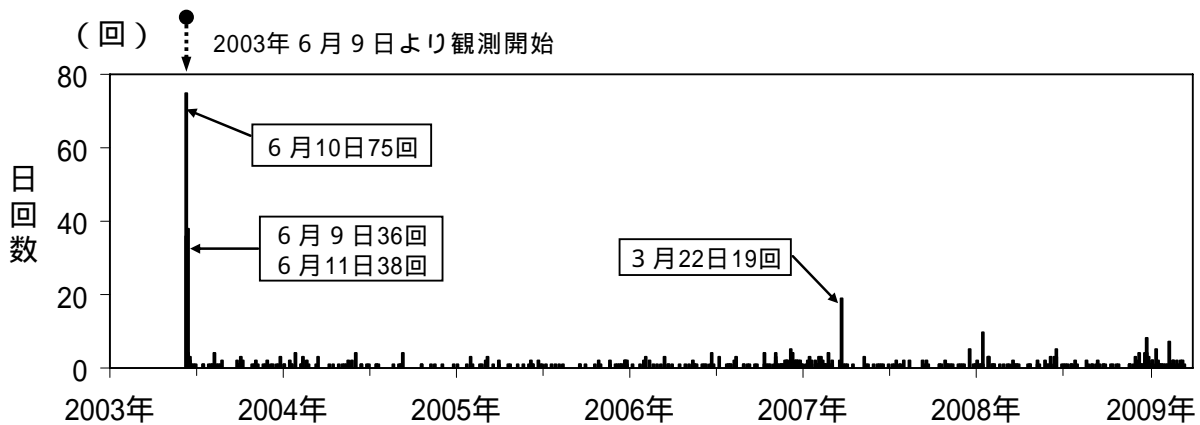
図 2 秋田駒ヶ岳 日別地震回数（2003 年 6 月 9 日～2009 年 3 月）
