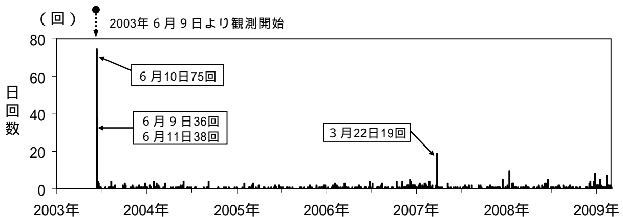
図 2 秋田駒ヶ岳 日別地震回数（2003 年 6 月 9 日～2009 年 2 月）
