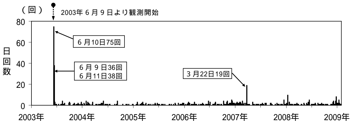
図 2 秋田駒ヶ岳 日別地震回数（2003 年 6 月 9 日～2009 年 1 月）
