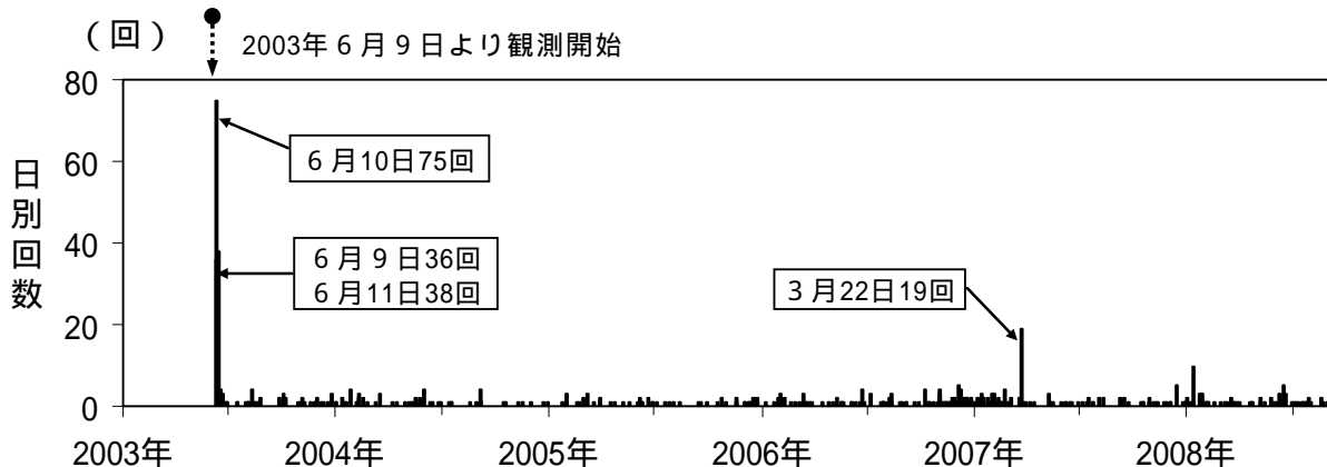
図 2 秋田駒ヶ岳 日別地震回数（2003 年 6 月 9 日～2008 年 8 月）
