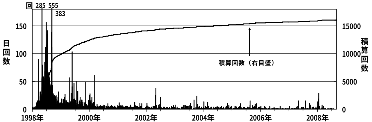
図 2※ 岩手山 日別地震回数（1998 年 1 月～2008 年 8 月）
