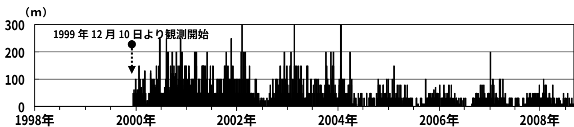
図 4 岩手山 日最大噴気の高さ（黒倉山）（1999 年 12 月 10 日～2008 年 8 月）
