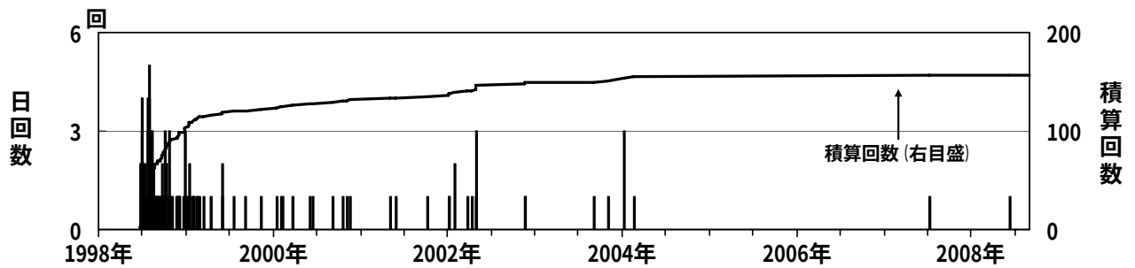
図 3※ 岩手山 日別微動回数（1998 年 1 月～2008 年 8 月）
