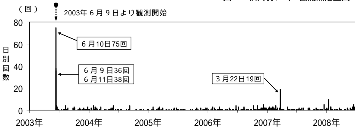
図 2 秋田駒ヶ岳 日別地震回数（2003 年 6 月 9 日～2008 年 6 月）
