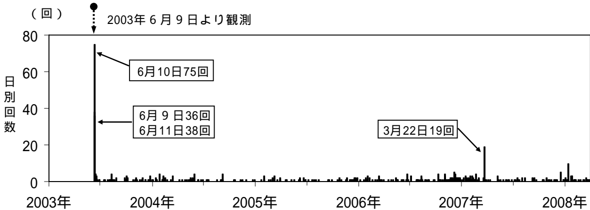
図 2 秋田駒ヶ岳 日別地震回数（2003 年 6 月 9 日～2008 年 3 月）
