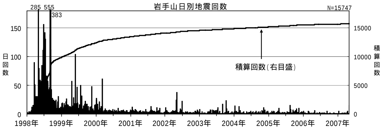
図 2 岩手山 日別地震回数(1998 年 1 月 ~ 2007 年 4 月)
