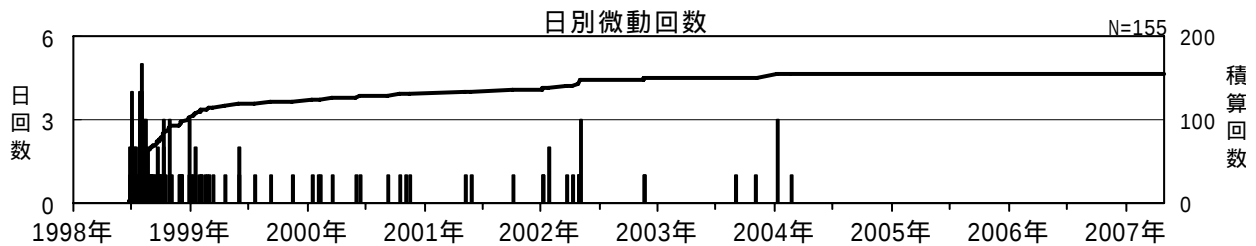
図 3 岩手山 日別微動回数(1998 年 1 月 ~ 2007 年 4 月)
