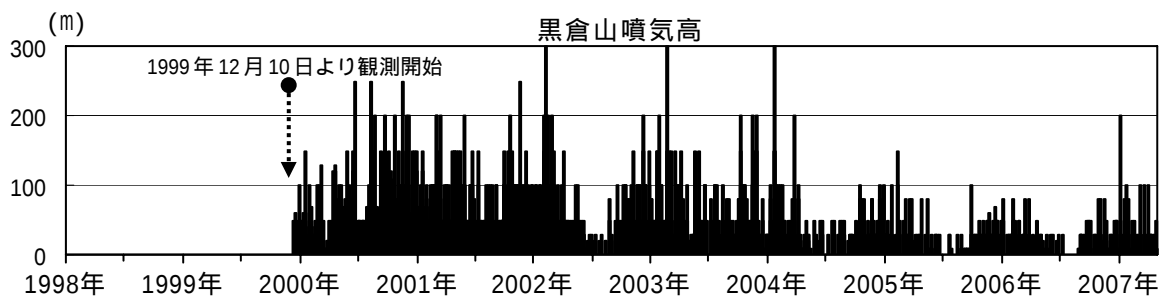
図 4 岩手山 日最大噴気の高さ（黒倉山）(1999 年 12 月 10 日 ~ 2007 年 4 月)
