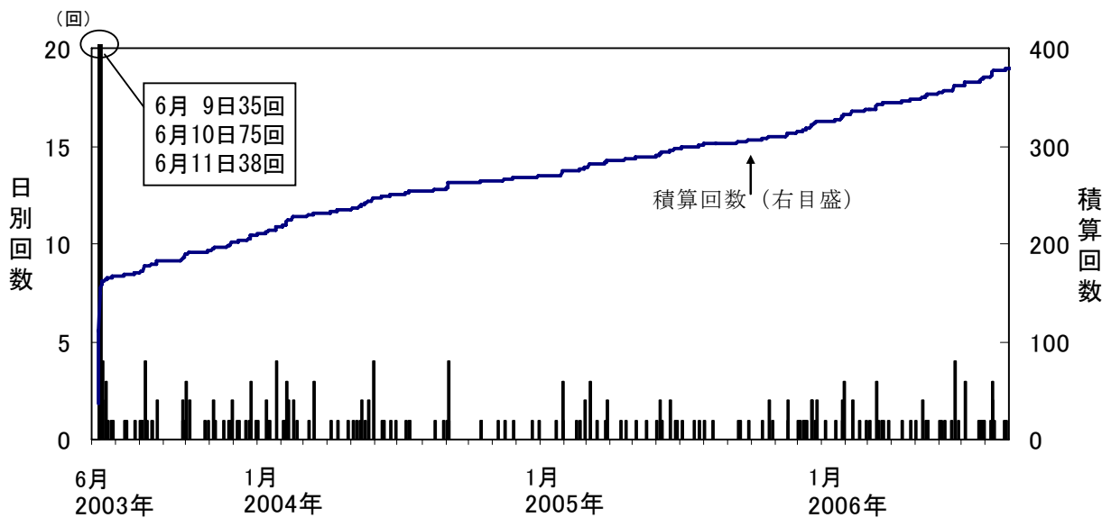
図2※ 秋田駒ヶ岳 日別地震回数（2003年6月9日～2006年8月）
