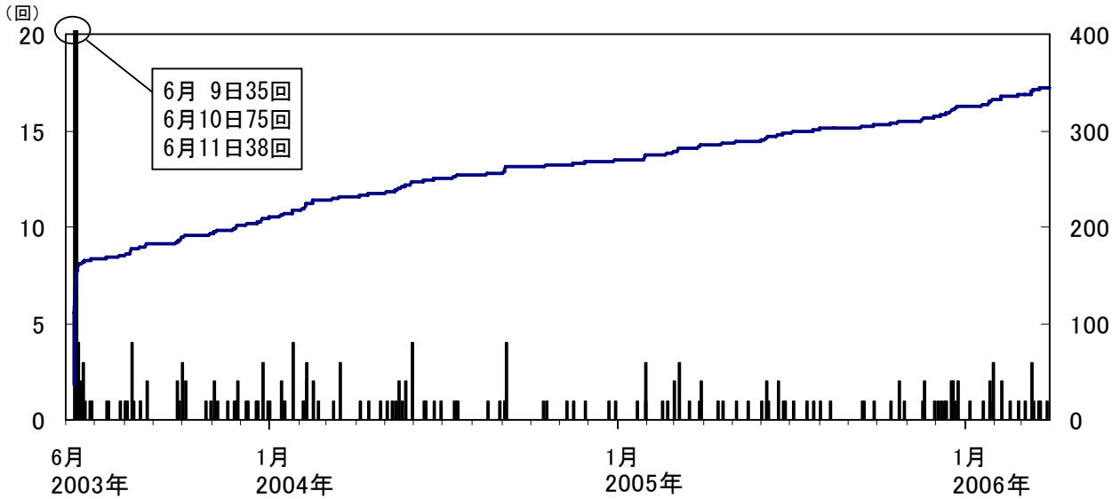
図2 ※ 秋田駒ヶ岳 日別地震回数（2003年6月9日～2006年3月）
