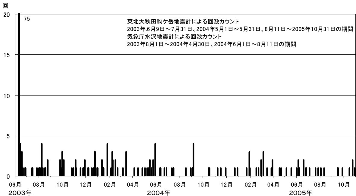
図2※ 秋田駒ヶ岳 日別地震回数（2003年6月9日～2005年10月31日）
