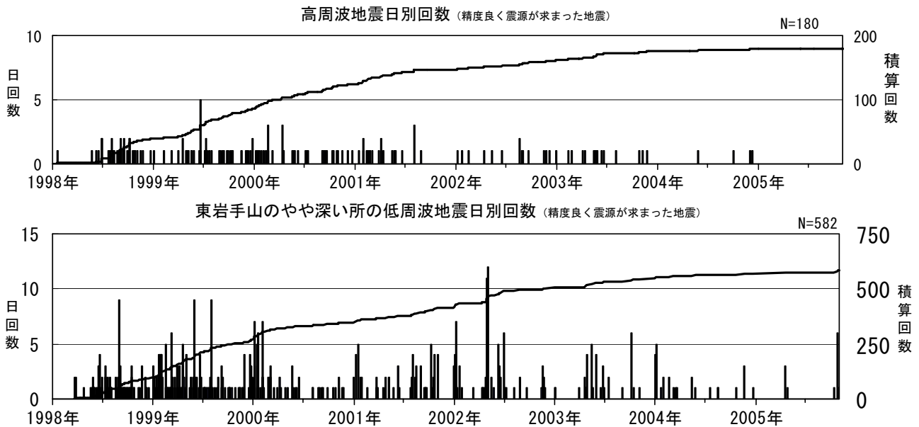
図3※ 岩手山 日別地震回数（1998年1月1日～2005年10月31日）
