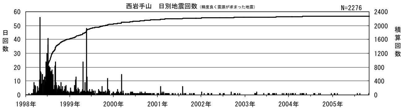
図4※ 東岩手山、西岩手山の日別地震回数 （1998年1月1日～2005年10月31日）
