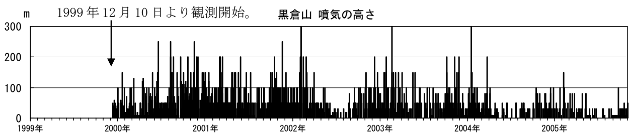
図2 岩手山 日最大噴気の高さ（黒倉山）
