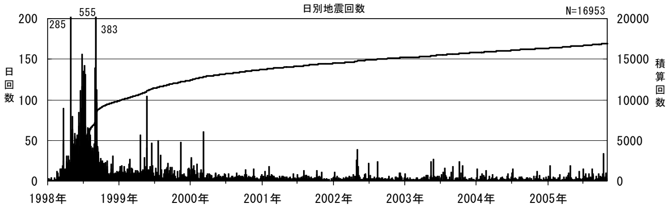
図3※ 岩手山 日別地震回数（1998年1月1日～2005年10月31日）
