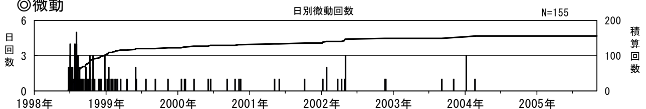
図5※ 岩手山 日別微動回数 （1998年1月1日～2005年10月31日）
