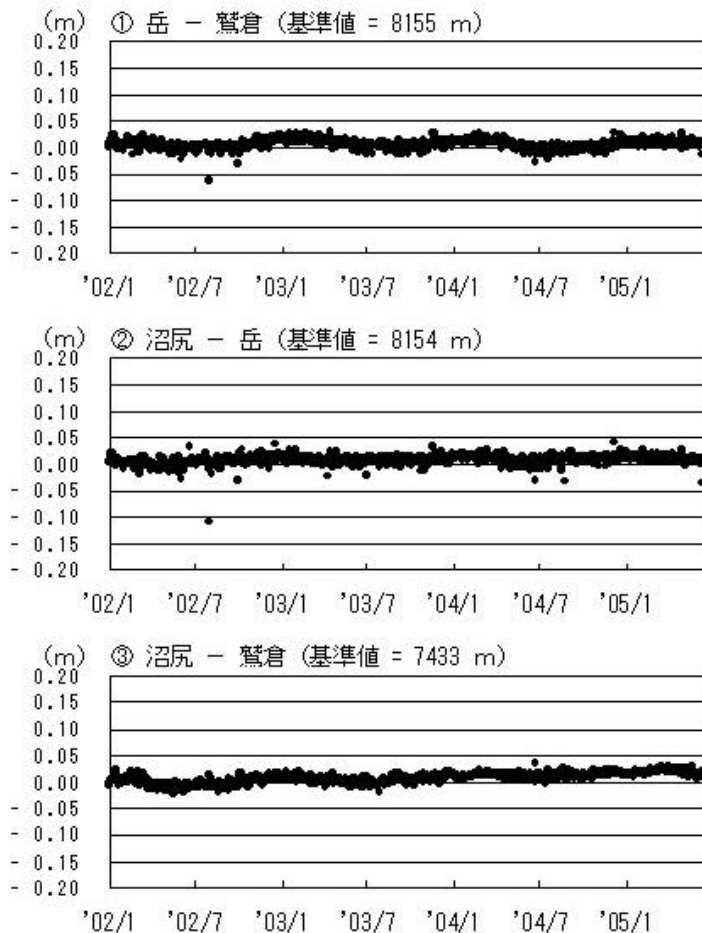
GPS 基線長変化図 (2002.1 ~ 2005.6)
