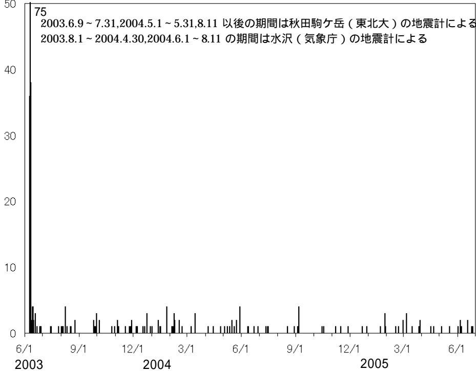
秋田駒ヶ岳日別地震回数
