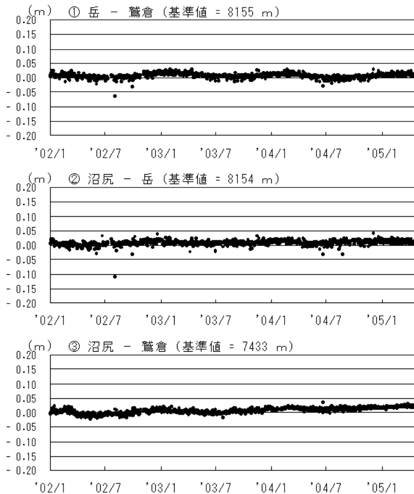
G P S 基線長変化図 (2002.1~2005.4)
