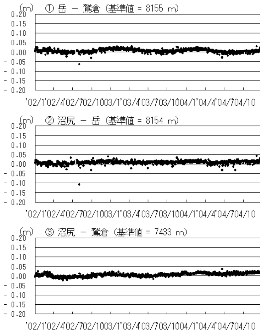
G P S 基線長変化図 (2002. 1~2004. 12)
