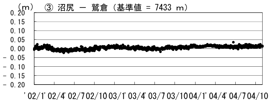
GPS 基線長変化図 (2002. 1~2004. 10)
