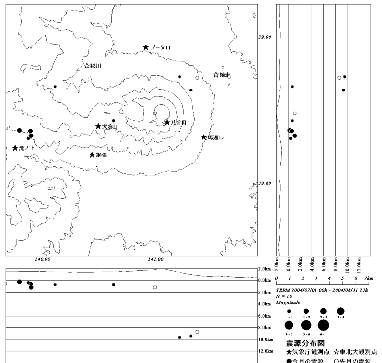
岩手山震源分布図(2004. 7. 1～2004. 8. 31)
