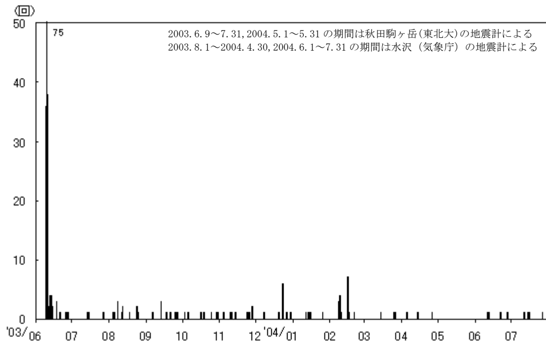
秋田駒ヶ岳日別地震回数(2003. 6. 9～2004. 7. 31)
