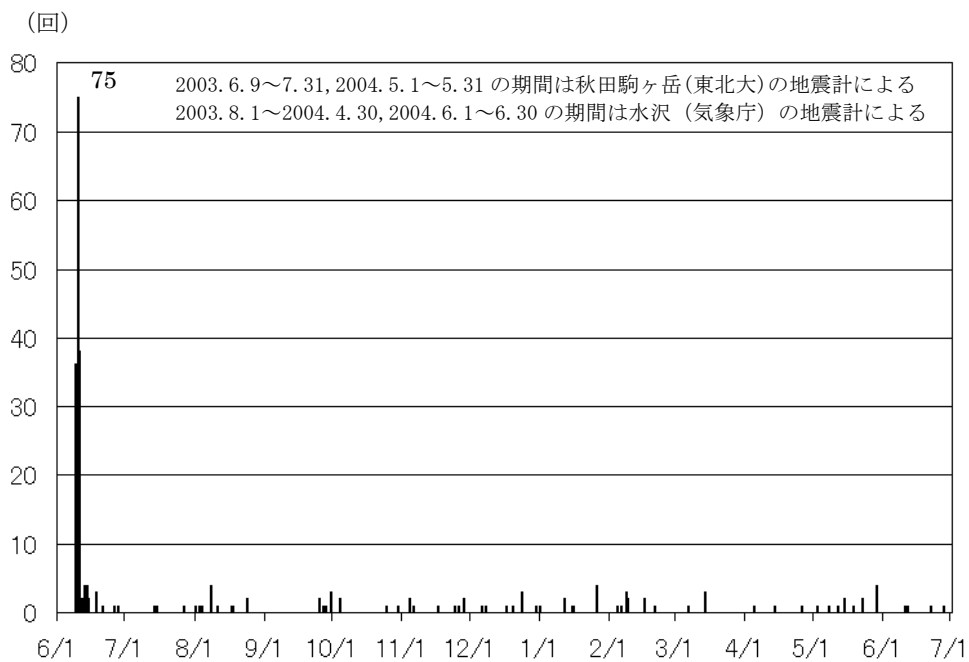
秋田駒ヶ岳日別地震回数
