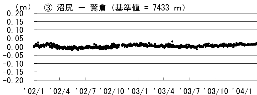
GPS 基線長変化図 (2002. 1 ~ 2004. 2)
