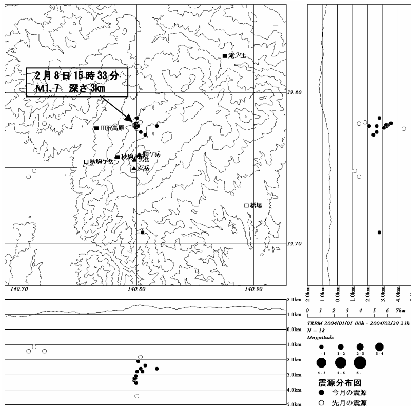
秋田駒ヶ岳震源分布図 (2004. 1. 1~2004. 2. 29)
