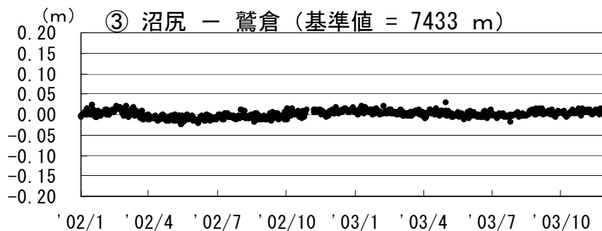
GPS 基線長変化図 (2002. 1~2003. 11)
