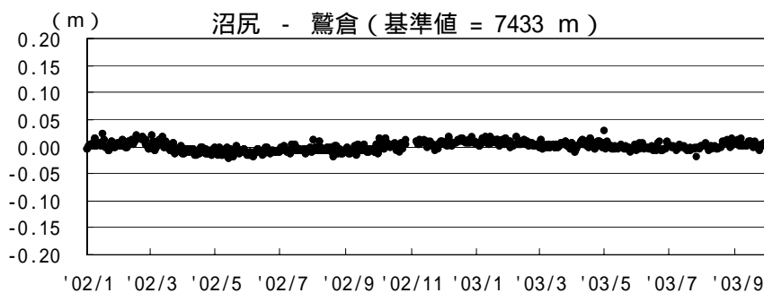
GPS 基線長変化図 (2002.1 ~ 2003.9)
