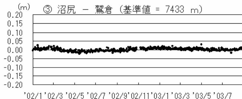
GPS 基線長変化図 (2002.01 ~ 2003.08)
