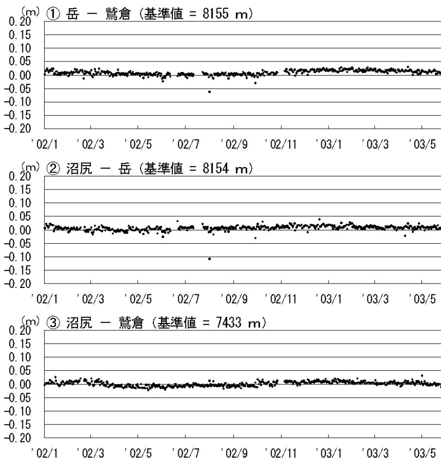
GPS 基線長変化図 (2002.01 ~ 2003.06)
