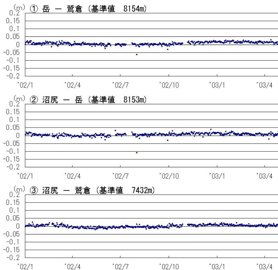
GPS 基線長変化図 (2002.01～2003.04)
