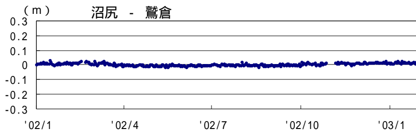
GPS 基線長変化図 (2002.01 ~ 2003.01)
