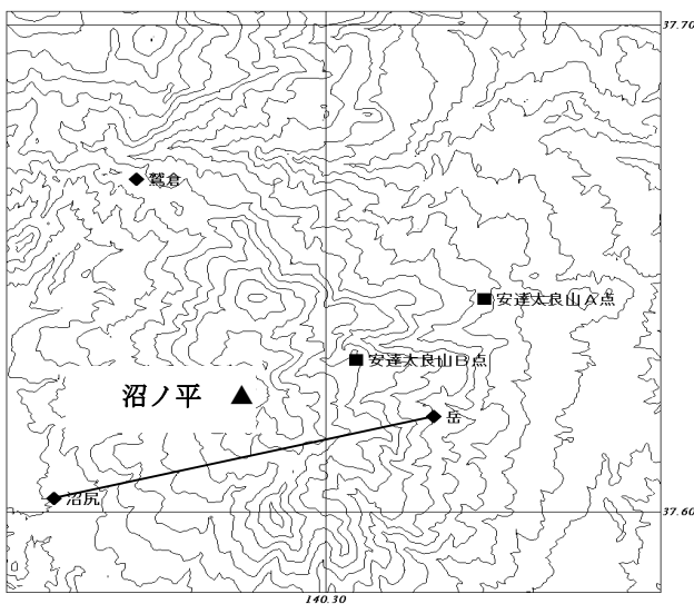
安達太良山観測点配置図
