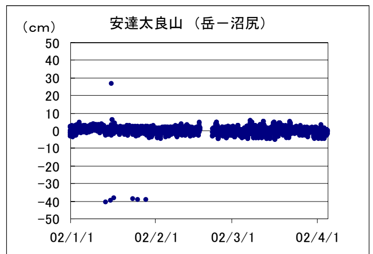
GPS基線長(2002.1~2002.3)
