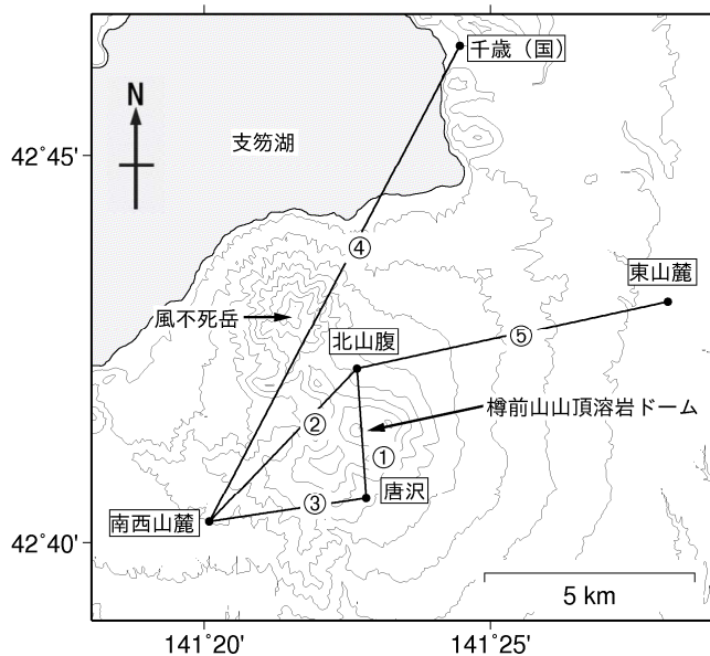
図5 樽前山 GNSS連続観測による基線長変化（2005年1月～2024年4月）及び観測点配置図
