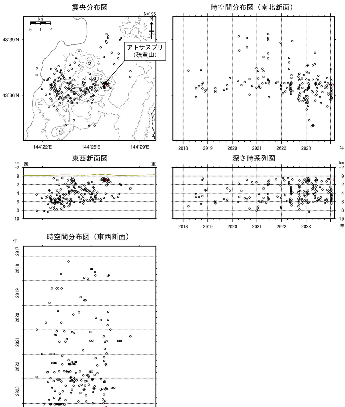
図3 アトサヌプリ 火山性地震の震源分布（2017年8月～2024年2月）
