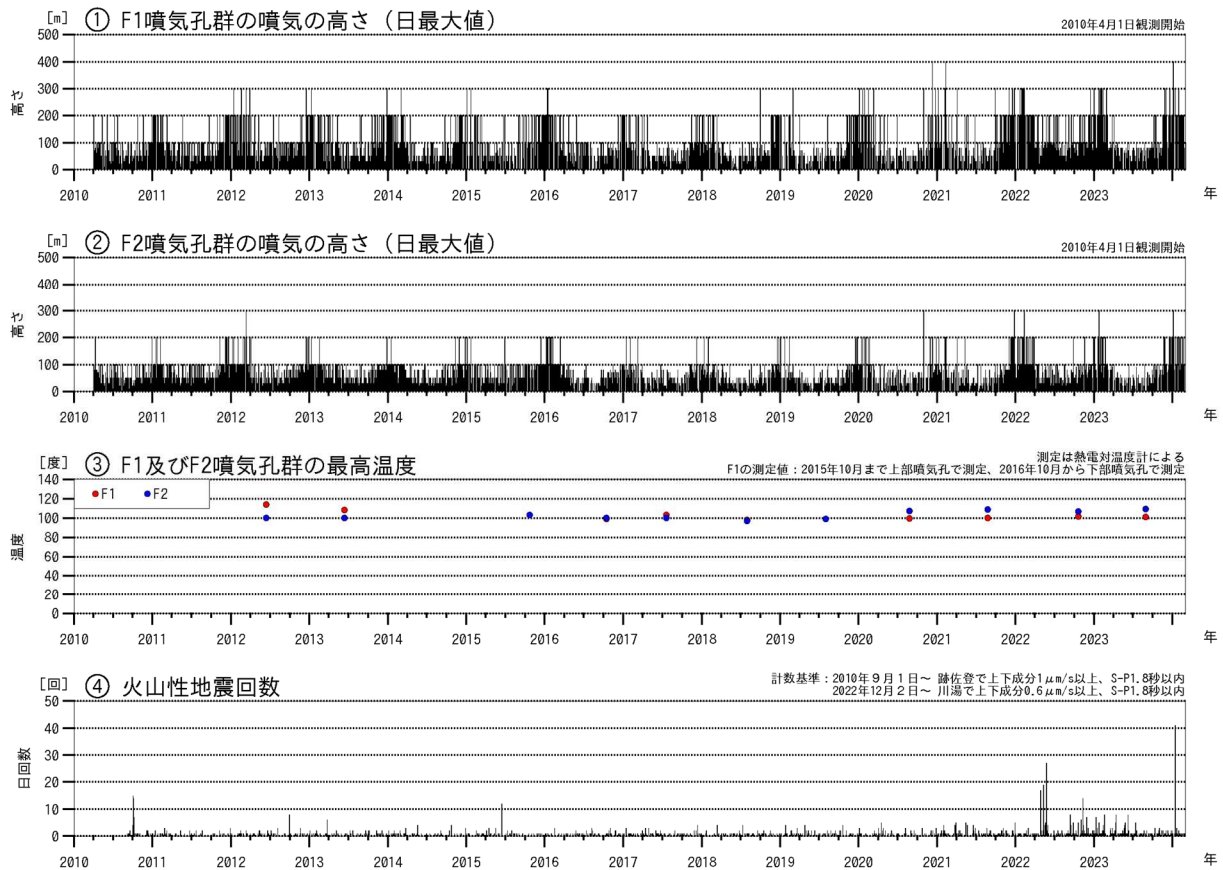
図1 アトサヌプリ 火山活動経過図 (2010年4月～2024年2月)
