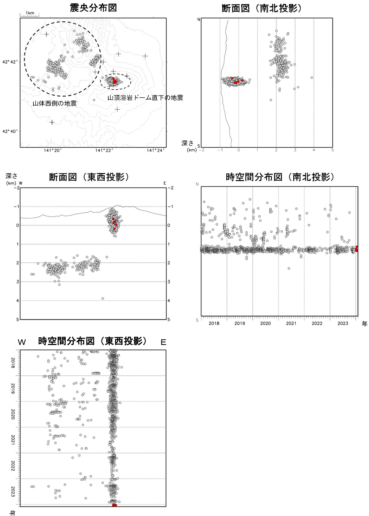
図3 樽前山 火山性地震の震源分布（2018年1月～2024年1月） ○：2018年1月～2023年12月の震源 ●：2024年1月の震源 +：地震観測点
