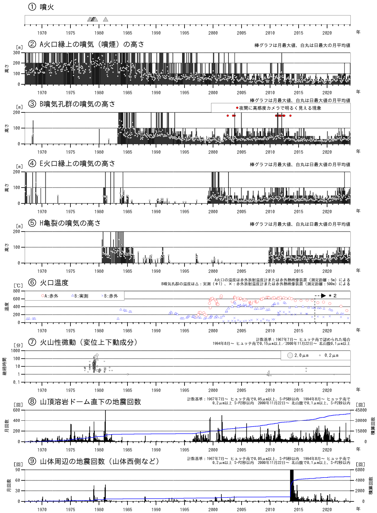
図2 樽前山 火山活動経過図（1967年1月～2024年1月）
