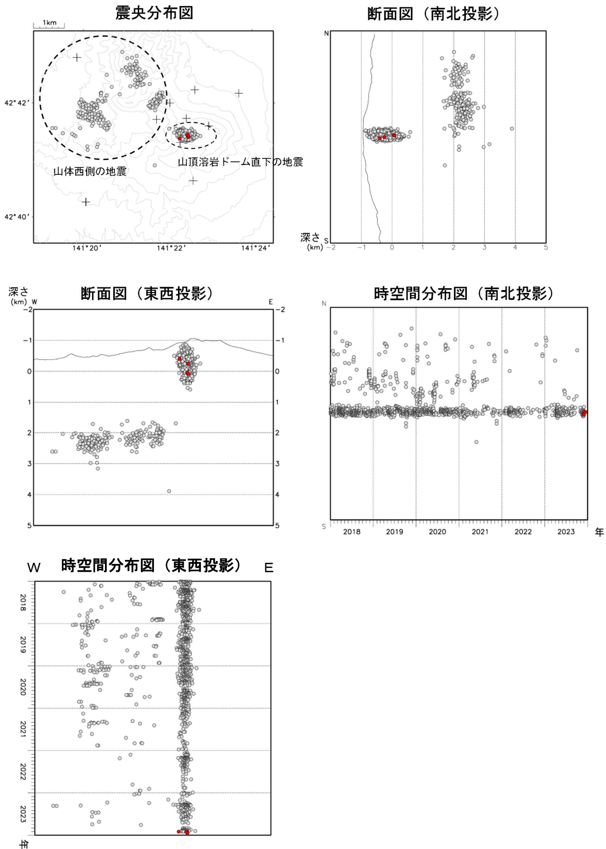
図3 樽前山 火山性地震の震源分布（2018年1月～2023年12月）
