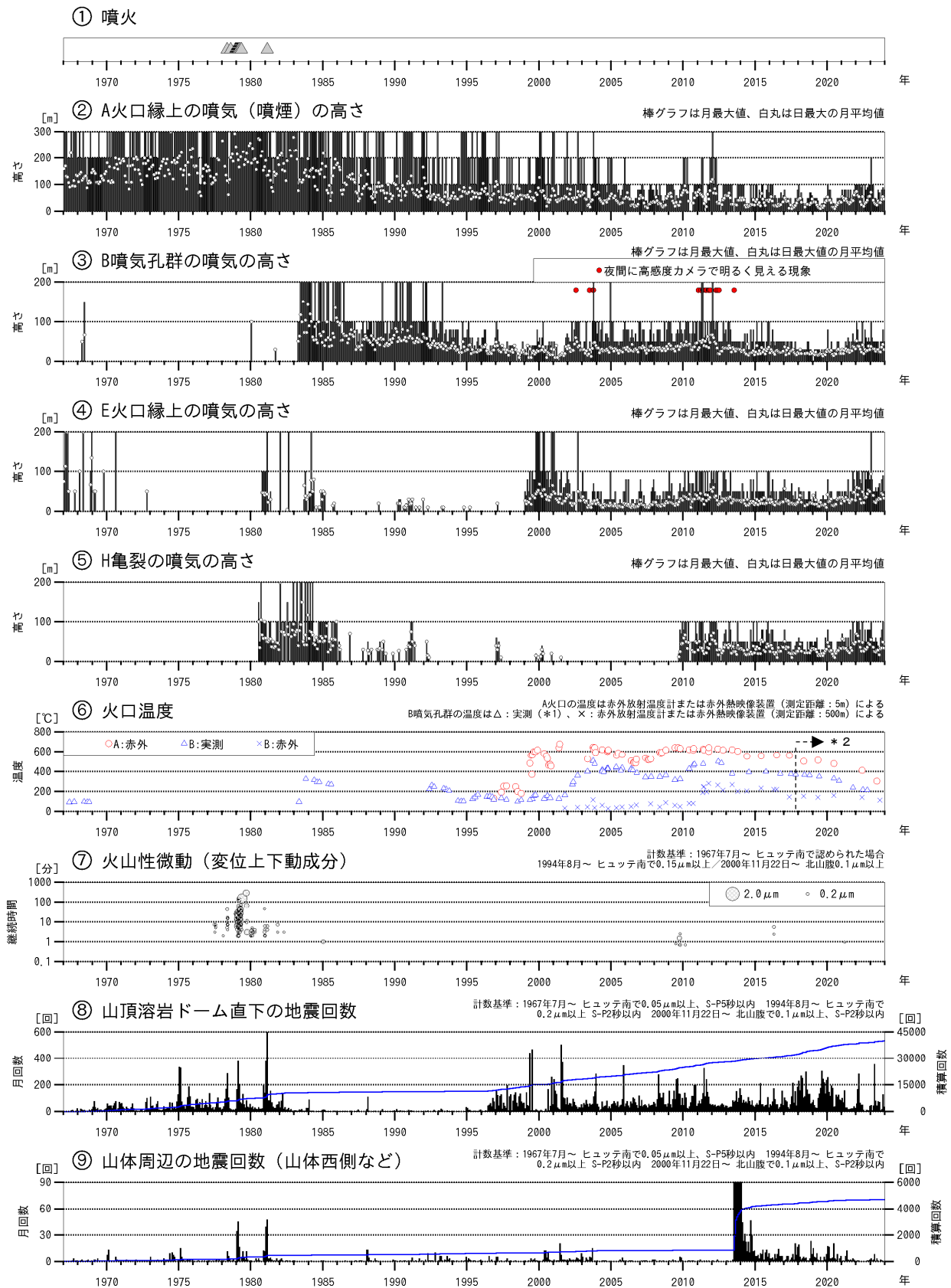
図2 樽前山 火山活動経過図(1967年1月~2023年12月)
