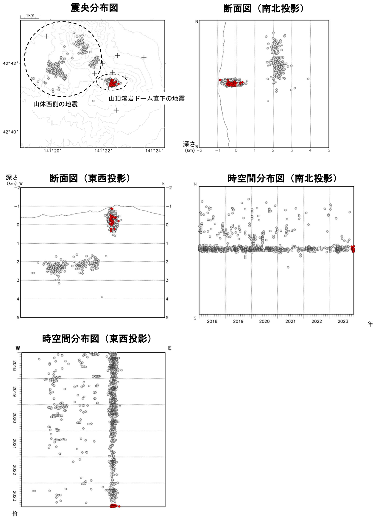
図3 樽前山 火山性地震の震源分布 (2018年1月~2023年11月)
