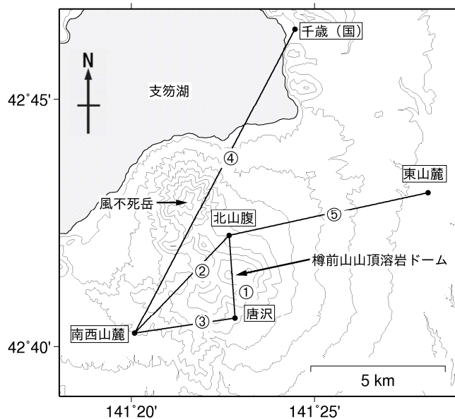
図4 樽前山 GNSS連続観測による基線長変化(2005年1月~2023年11月)及び観測点配置図 グラフ①~⑤は観測点配置図の基線①~⑤に対応しています。 グラフ中の空白部分は欠測を示しています。 ②~④の楕円内の変動(*1)は2014年7月8日に発生した胆振地方中東部の地震によるものです。
