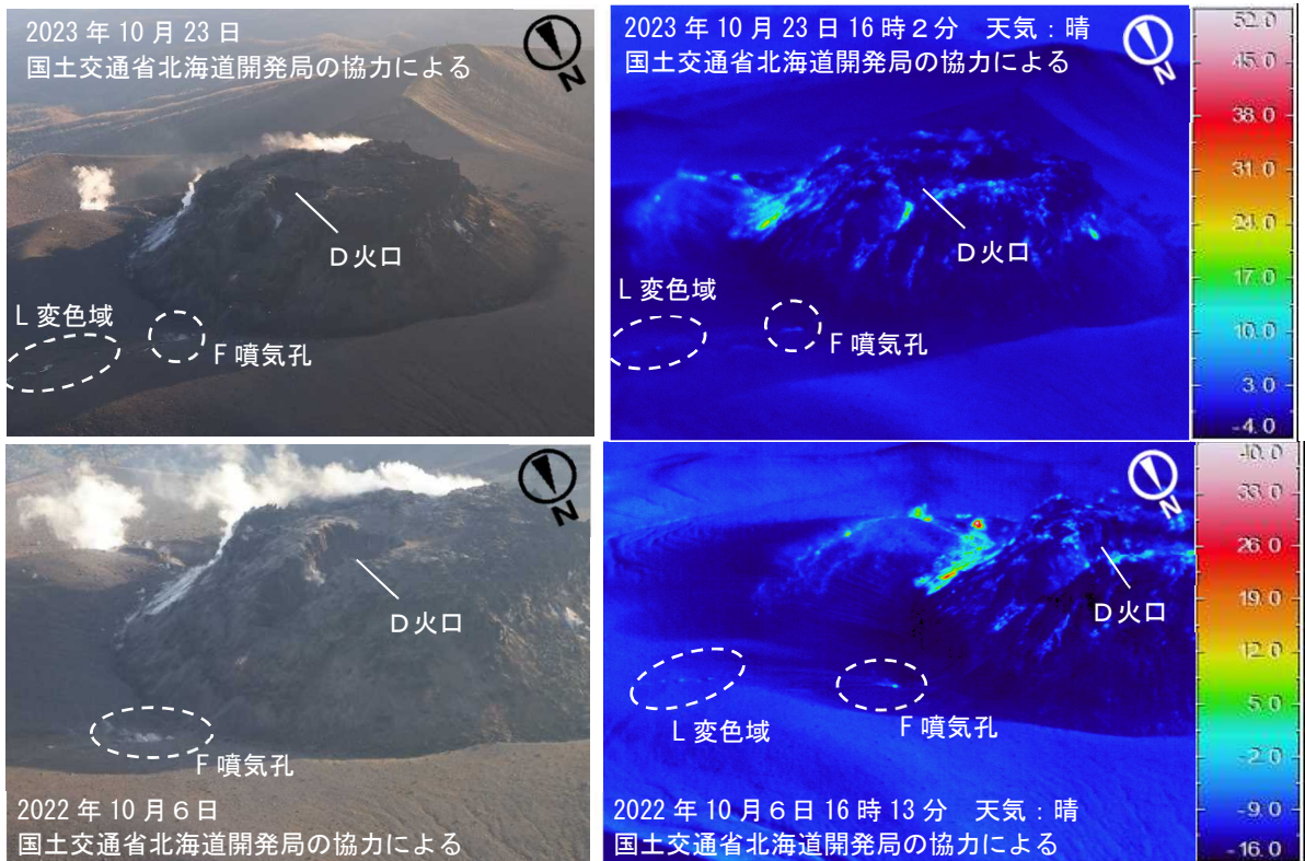
図4 樽前山 赤外熱映像装置による山頂溶岩ドーム北側～北東側の地表面温度分布 上：北東側上空（図3の①）から撮影 下：北東側上空（図3の②）から撮影 ・前回の観測（2022年10月）と比較して、山頂溶岩ドームの地表面温度分布の状況に変化は認められませんでした。
