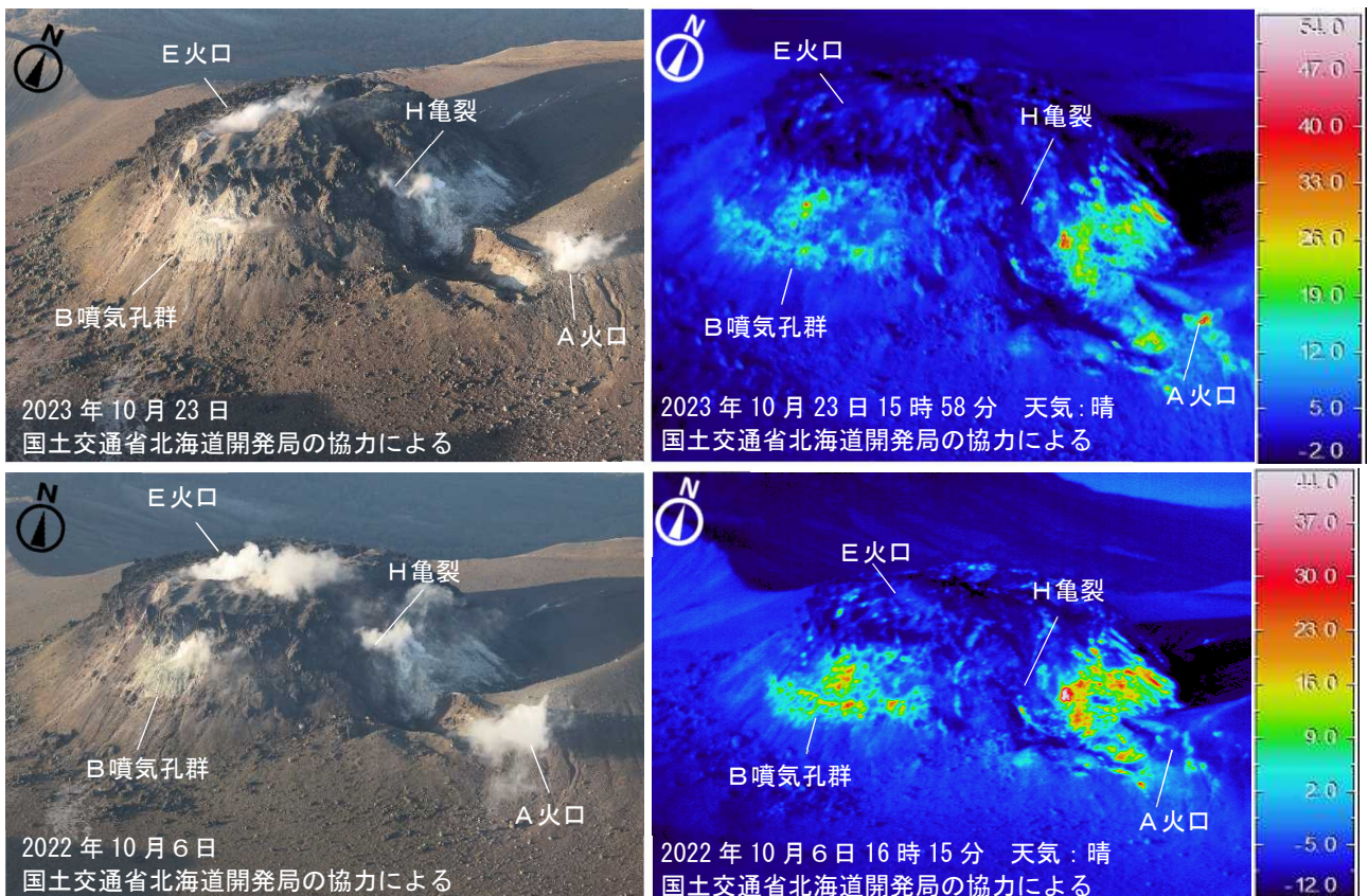
図5 樽前山 赤外熱映像装置による山頂溶岩ドーム南側～南東側の地表面温度分布 上：南側上空（図3の③）から撮影 下：南側上空（図3の④）から撮影 ・前回の観測（2022年10月）と比較して、山頂溶岩ドームの地表面温度分布の状況に変化は認められませんでした。前回観測でA火口付近の温度は噴気の影響を受けていた可能性があります。
