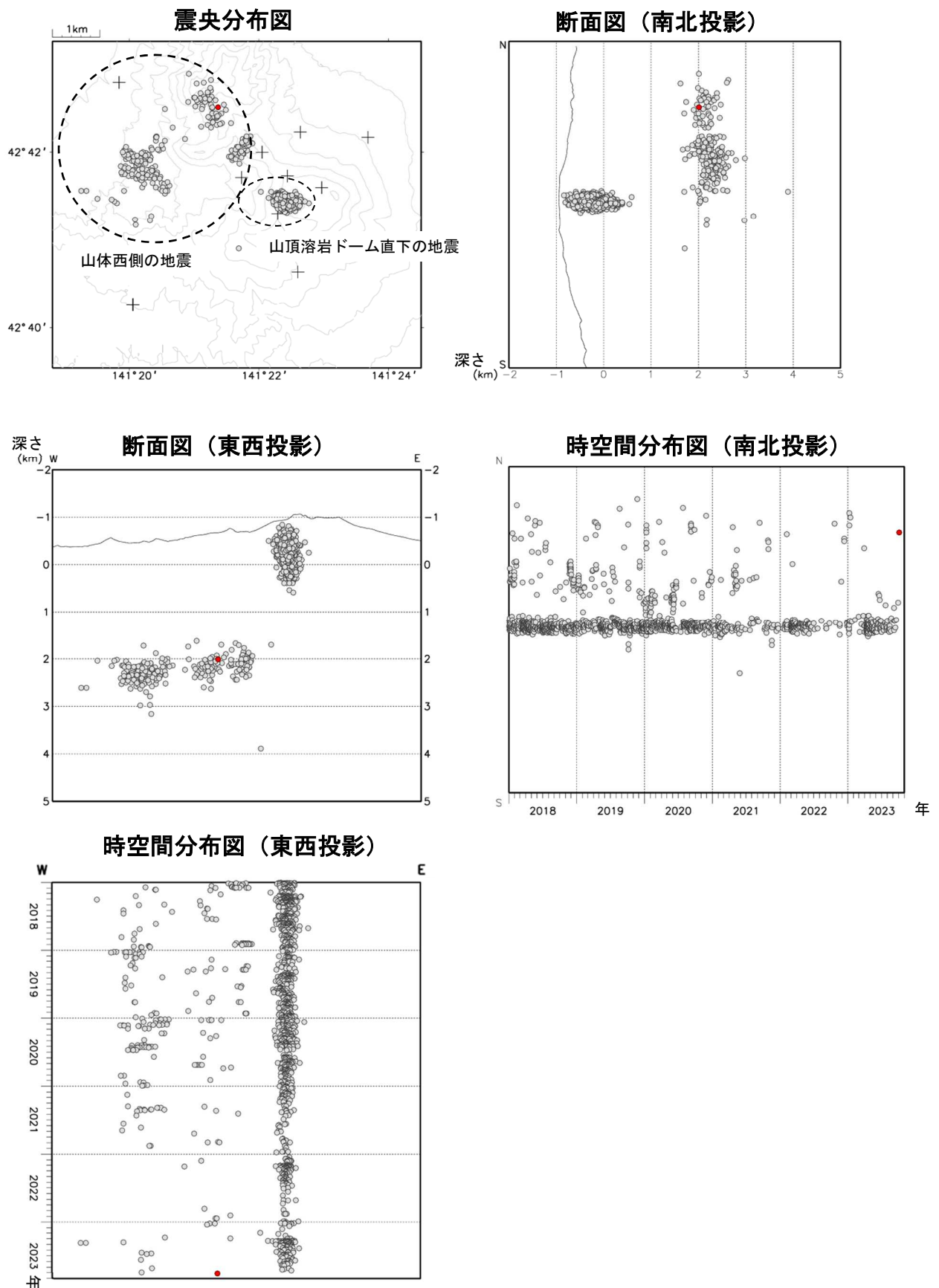
図6 樽前山 火山性地震の震源分布（2018年1月～2023年10月）
