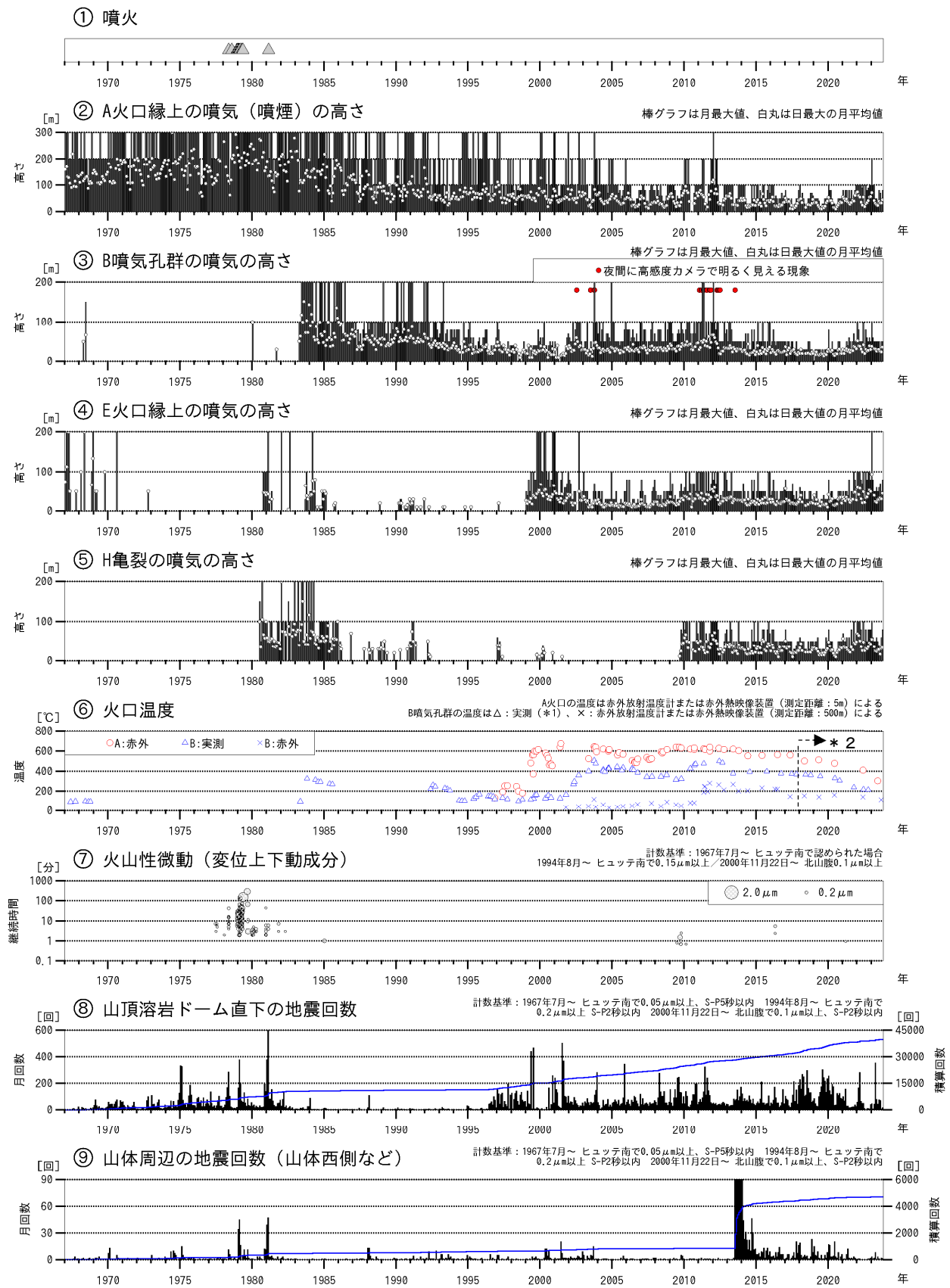
図1 樽前山 火山活動経過図（1967年1月～2023年10月）
