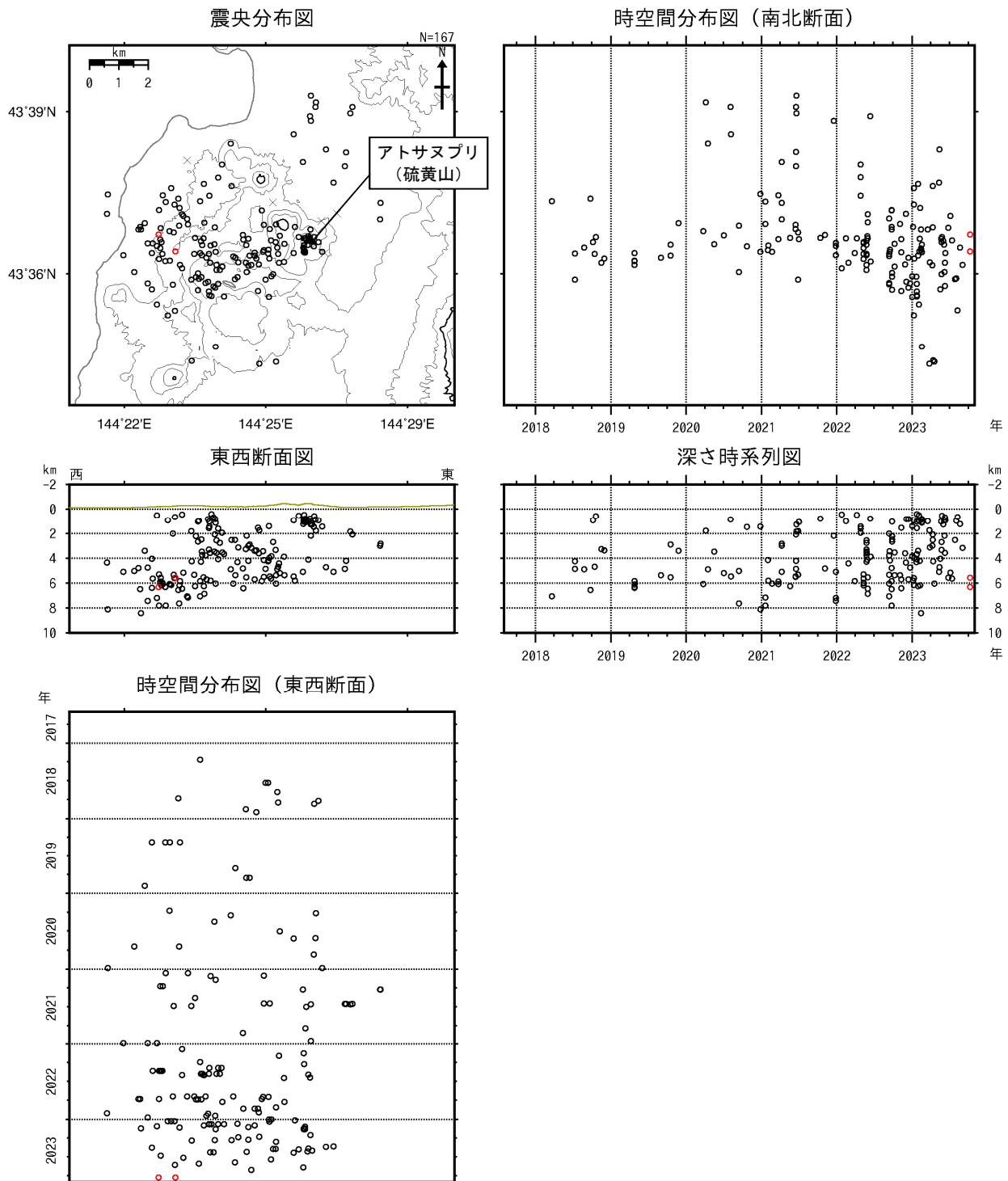
図3 アトサヌプリ 火山性地震の震源分布（2017年8月～2023年10月）
