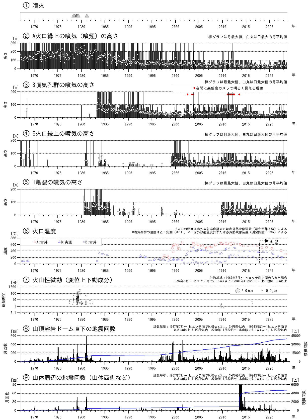
図2 樽前山 火山活動経過図(1967年1月~2023年9月)
