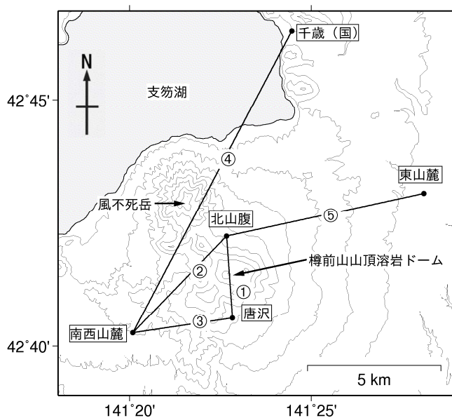
図4 樽前山 GNSS連続観測による基線長変化(2005年1月~2023年9月)及び観測点配置図 グラフ①~⑤は観測点配置図の基線①~⑤に対応しています。 グラフ中の空白部分は欠測を示しています。 ②~④の楕円内の変動(*1)は2014年7月8日に発生した胆振地方中東部の地震によるものです。
