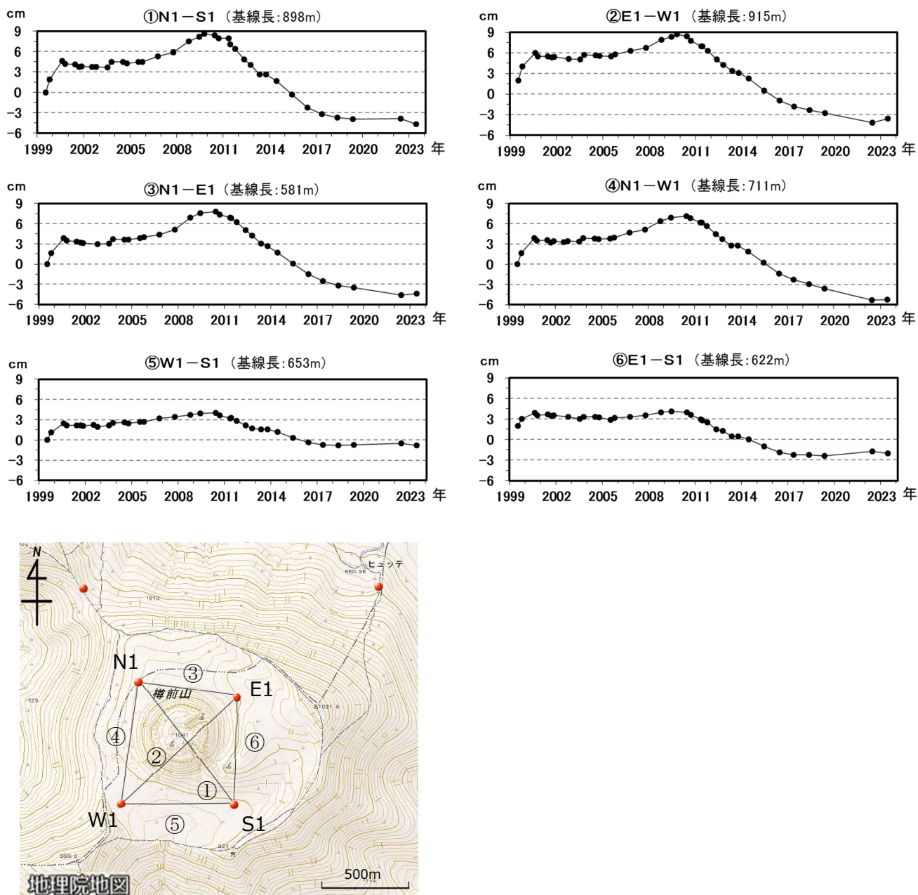
図4 樽前山 GNSS 繰り返し観測による基線長変化（1999年～2023年）及び観測点配置図と基線組み合わせ
