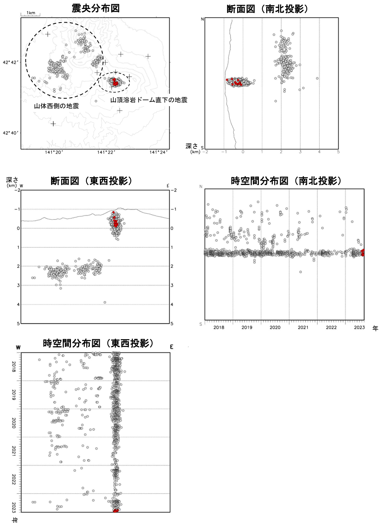
図3 樽前山 火山性地震の震源分布（2018年1月～2023年8月） ○：2018年1月～2023年7月の震源 ●：2023年8月の震源 +：地震観測点
