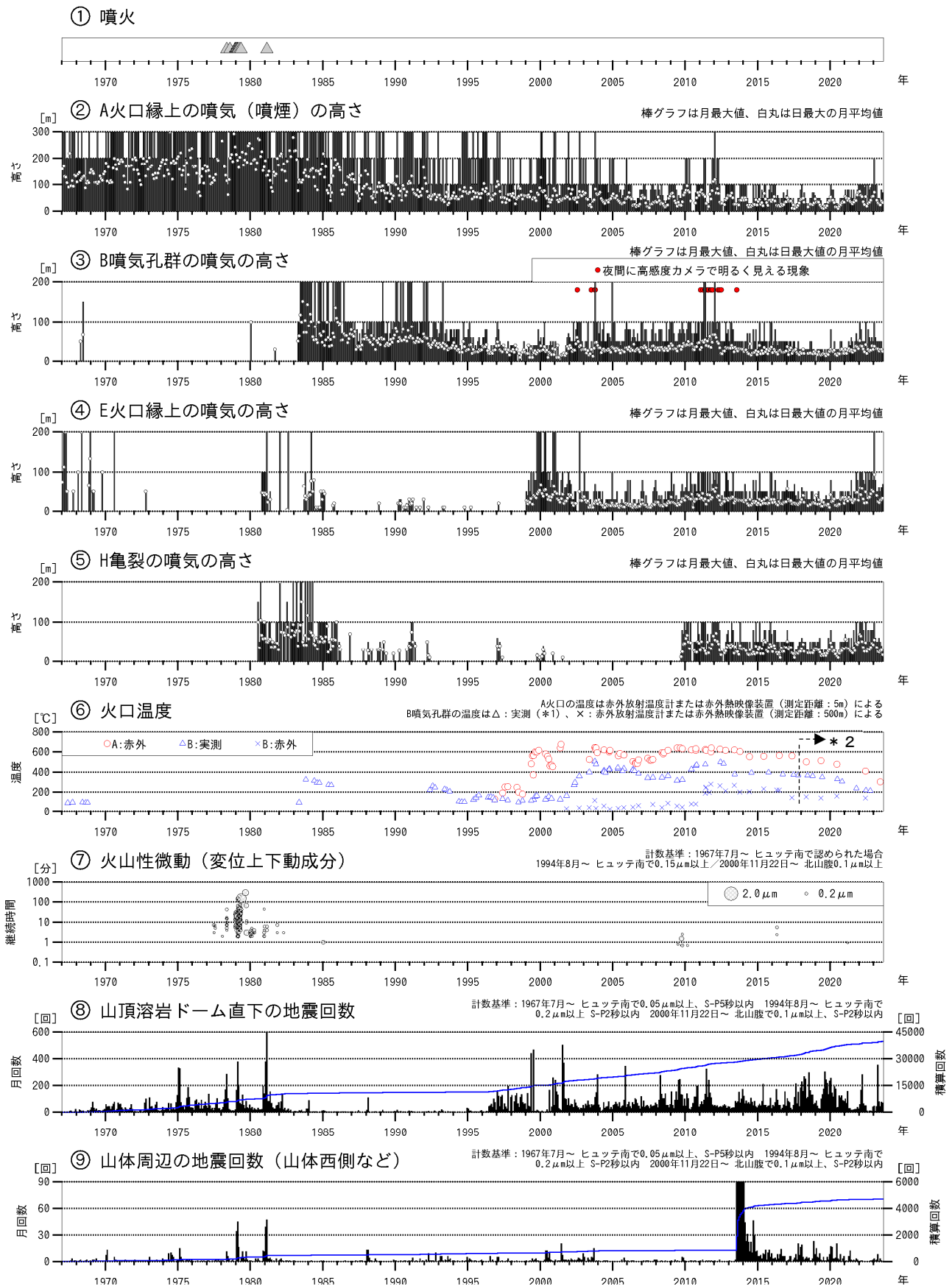
図2 樽前山 火山活動経過図(1967年1月~2023年8月)
