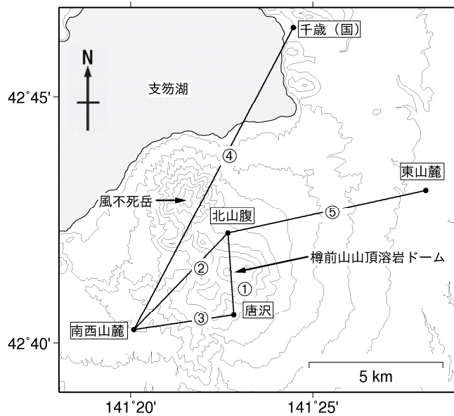
図6 樽前山 GNSS連続観測による基線長変化（2005年1月～2023年6月）及び観測点配置図 グラフ①～⑤は観測点配置図の基線①～⑤に対応しています。 グラフ中の空白部分は欠測を示しています。 ②～④の楕円内の変動（*1）は2014年7月8日に発生した胆振地方中東部の地震によるものです。
