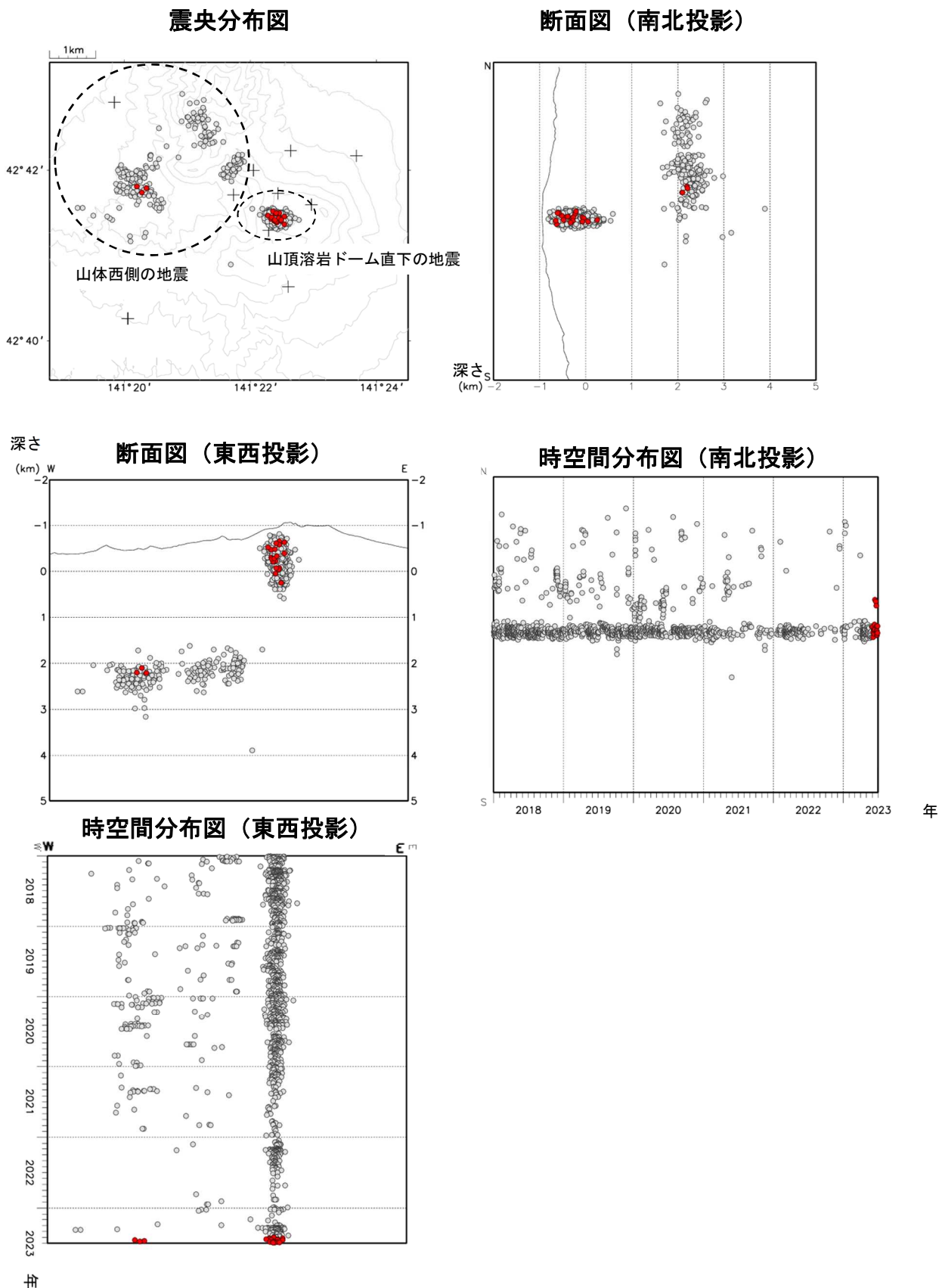
図5 樽前山 火山性地震の震源分布（2018年1月～2023年6月） ○：2018年1月～2023年5月の震源 ●：2023年6月の震源 +：地震観測点
