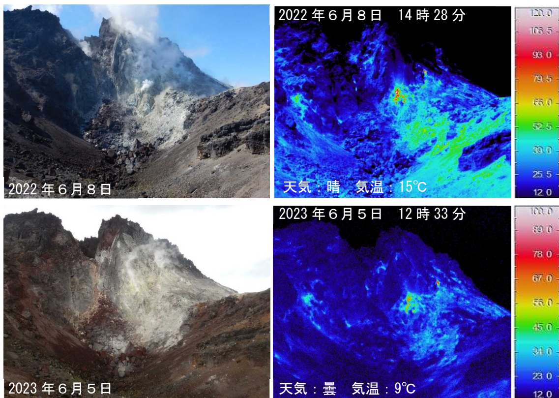
図4 樽前山 赤外熱映像装置によるH亀裂の地表面温度分布の比較
