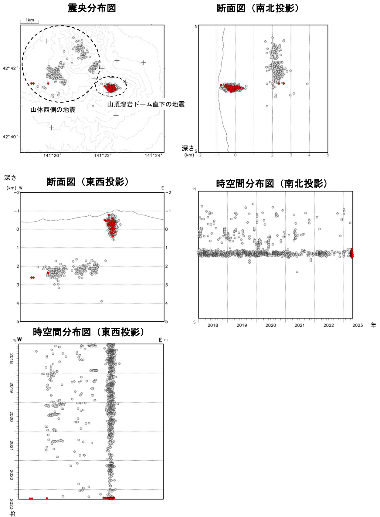
図3 樽前山 火山性地震の震源分布 (2018年1月~2023年4月) ○ : 2018年1月~2023年3月の震源 ● : 2023年4月の震源 + : 地震観測点
