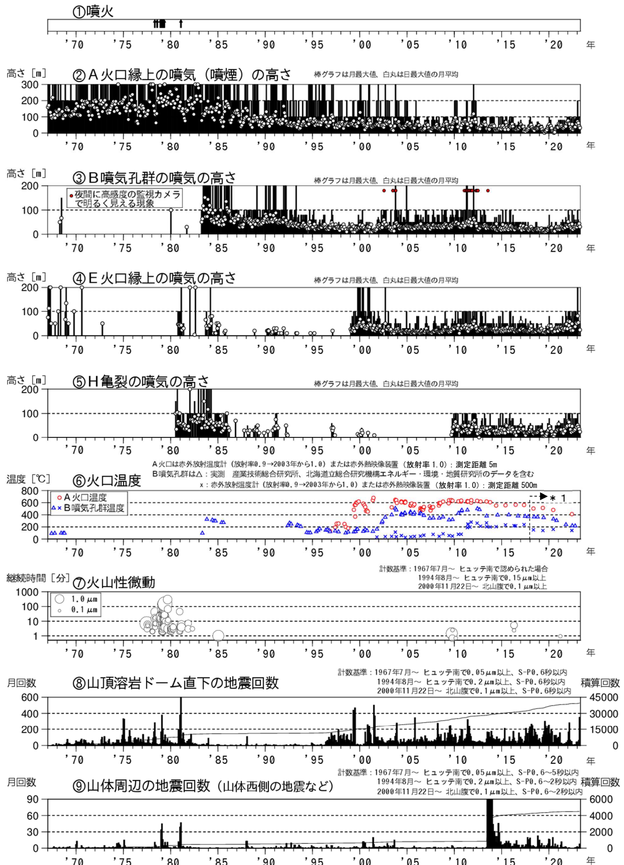
図2 樽前山 火山活動経過図(1967年1月~2023年4月)
