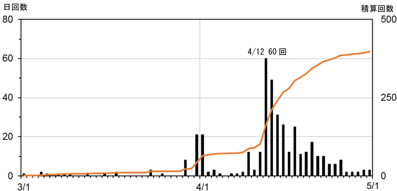
図4 樽前山 山頂溶岩ドーム直下の地震回数の推移（2023年3月～2023年4月） ・ドーム直下浅部の領域では3月下旬から振幅の小さな火山性地震がやや増加し始め、4月12日には一時的に増加して60回を数えましたが、その後は次第に減少し、下旬には1日あたり数回以下となりました。
