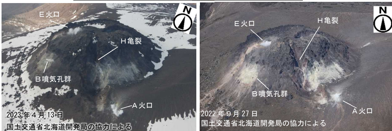
図5 樽前山 山頂溶岩ドーム南側～南東側の噴気の様子 左：南側上空（上図の①）から撮影 右：南側上空（上図の②）から撮影 ・前回の観測（2022年9月）と比較して、噴気等の様子に変化は認められませんでした。
