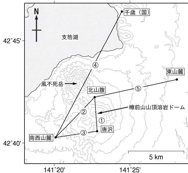
図6 樽前山 GNSS連続観測による基線長変化（2005年1月～2023年4月）及び観測点配置図
