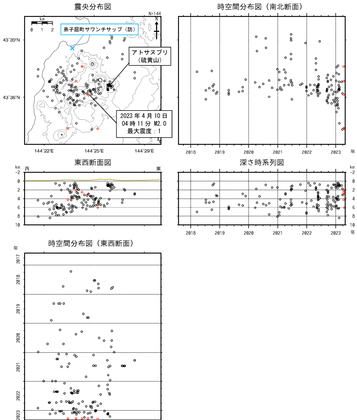
図3 アトサヌプリ 火山性地震の震源分布（2017年8月～2023年4月）
