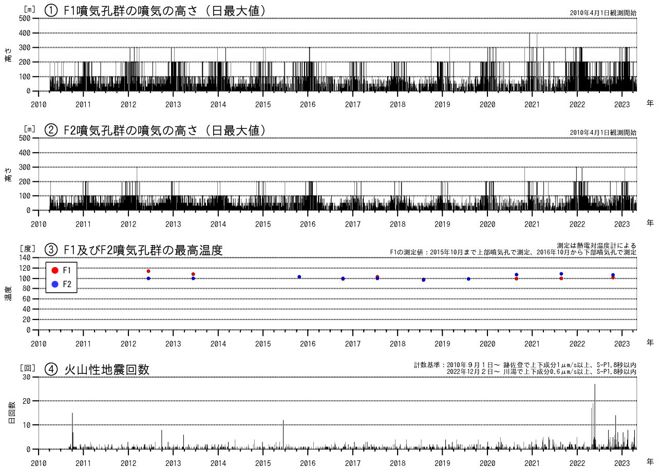
図1 アトサヌプリ 火山活動経過図（2010年4月～2023年4月）
