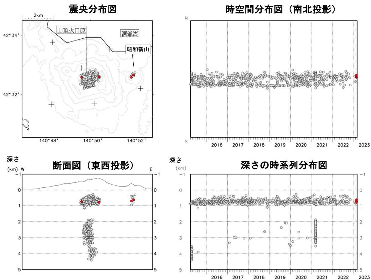
図3 有珠山 火山性地震の震源分布（2015年4月～2023年2月）
