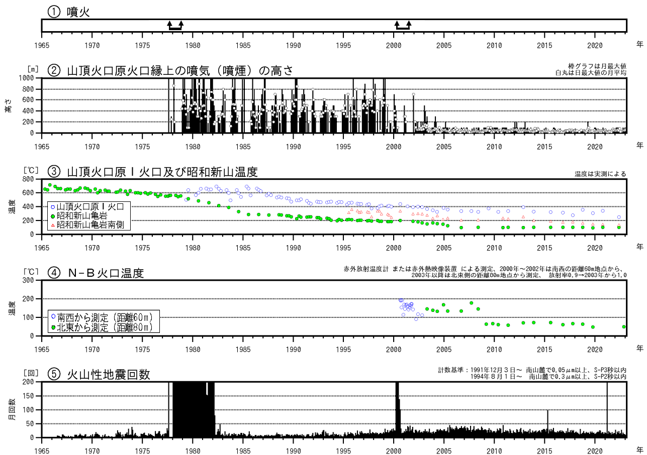
図1 有珠山 火山活動経過図（1965年1月～2023年2月）
