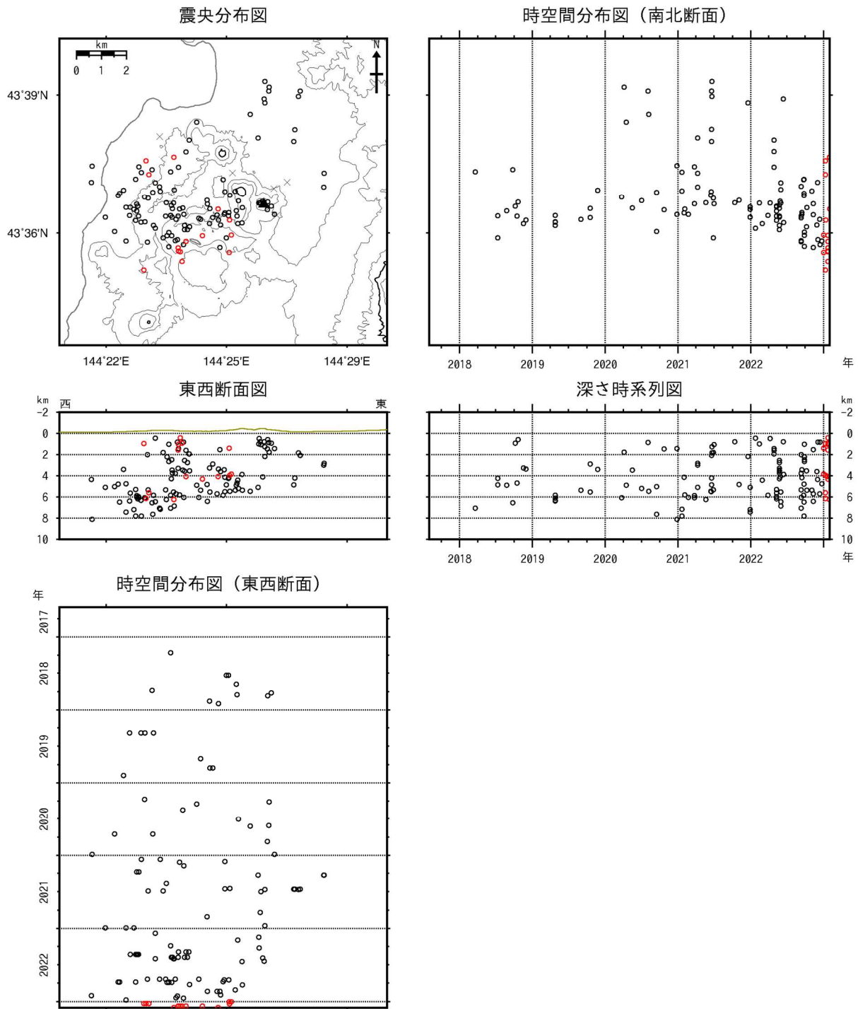
図3 アトサヌプリ 火山性地震の震源分布（2017年8月～2023年1月）
