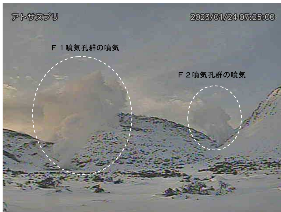
図2 アトサヌプリ 北側から見たF 1 噴気孔群及びF 2 噴気孔群の状況 （硫黄山駐車場北監視カメラによる）
