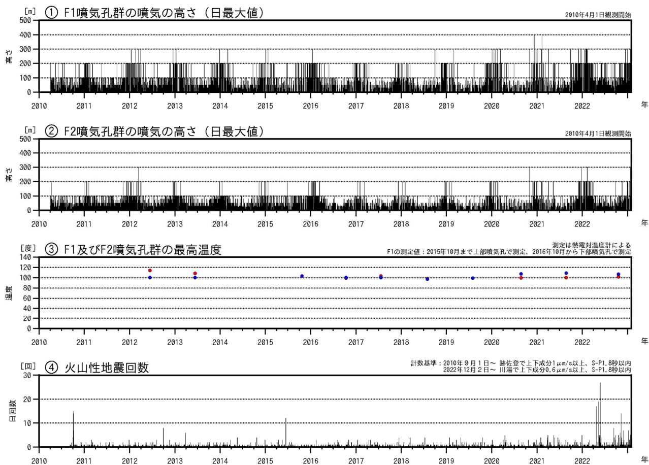
図1 アトサヌプリ 火山活動経過図（2010年4月～2023年1月）
