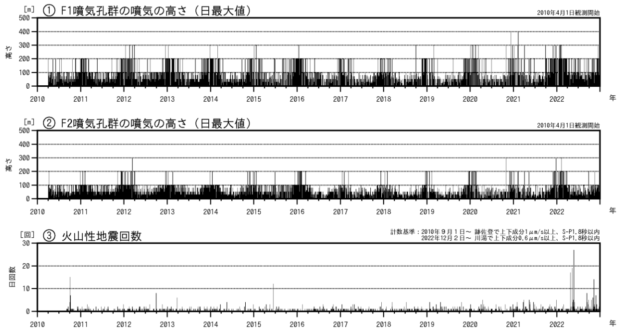
図1 アトサヌプリ 火山活動経過図（2010年4月～2022年12月）
