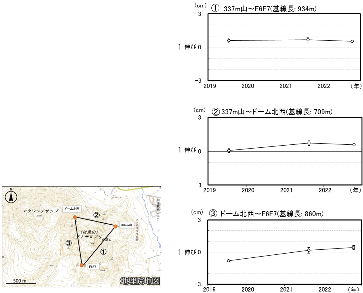
図5 アトサヌプリ GNSS繰り返し観測による基線長変化及び観測点配置図 (2019年8月～2022年10月) GNSS基線①～③は観測点配置図の①～③に対応しています。 ・前回の観測 (2021年8月) に比べて、特段の変化は認められませんでした。
