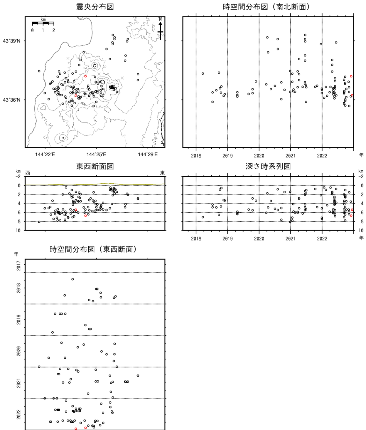
図3 アトサヌプリ 火山性地震の震源分布（2017年8月～2022年12月）
