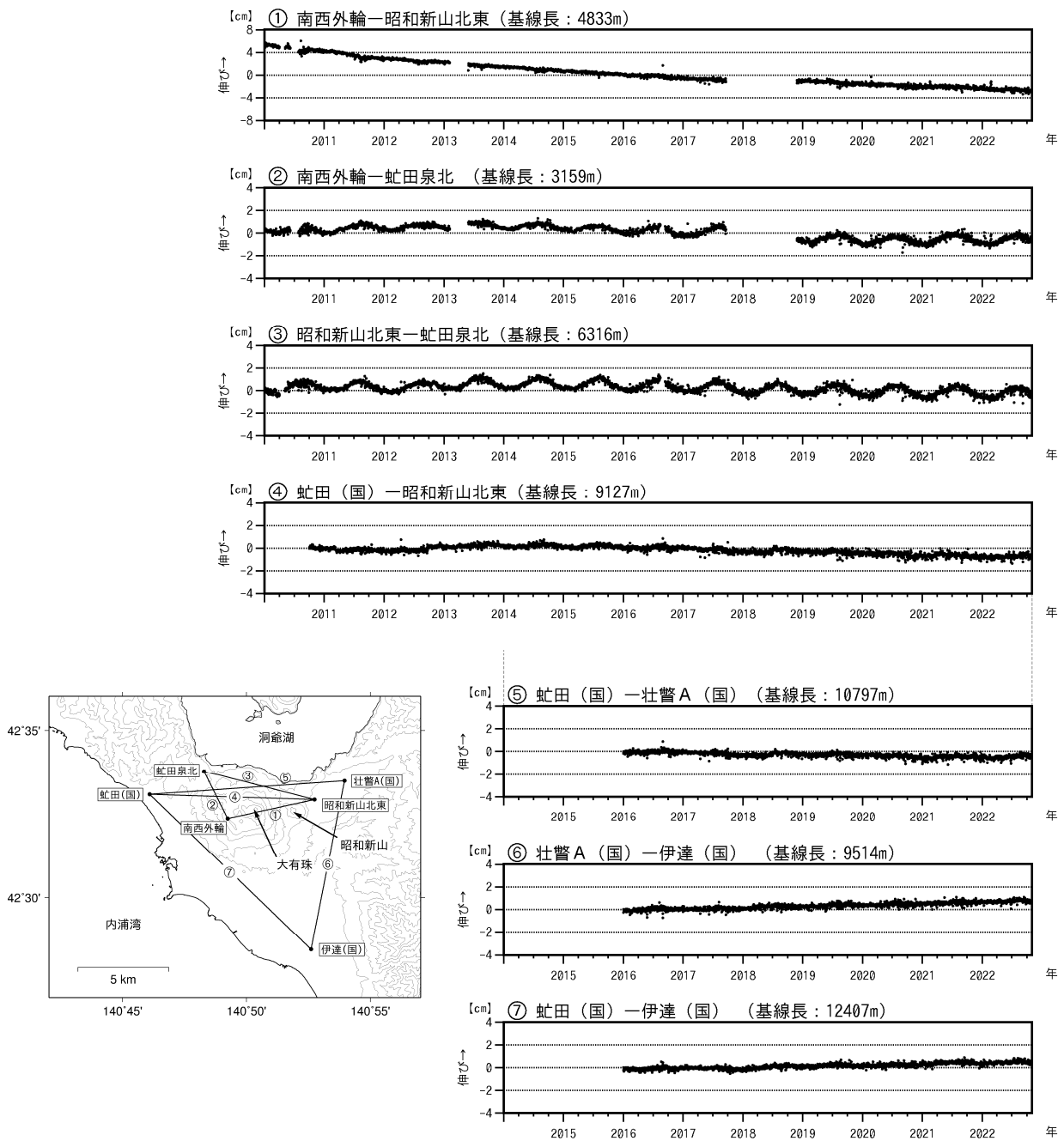
図6 有珠山 GNSS連続観測による基線長変化（2010年1月～2022年11月）及び観測点配置図 グラフ①～⑦は観測点配置図の基線①～⑦に対応しています。 グラフの空白部分は欠測を示します。
