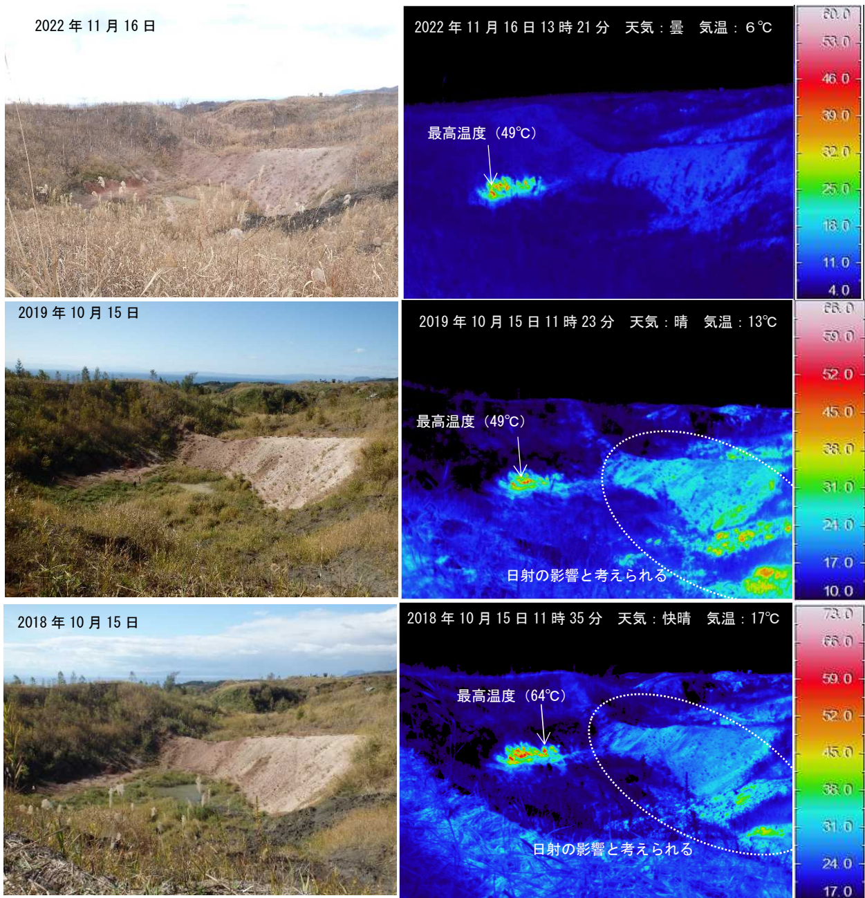
図3 有珠山 赤外熱映像装置によるN-B火口の地表面温度分布
