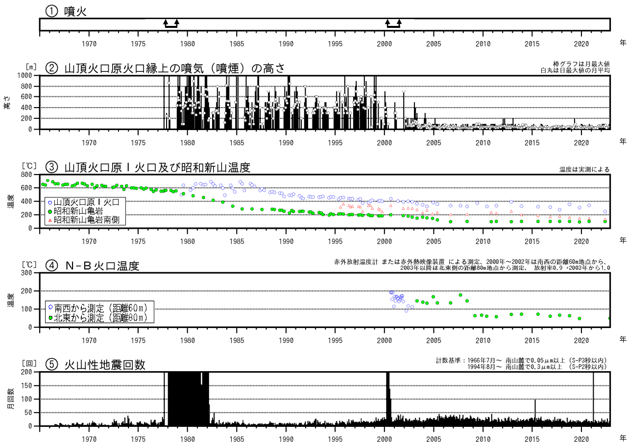
図1 有珠山 火山活動経過図（1965年1月～2022年11月） ↑印で挟まれた期間は噴火活動期を示します。
