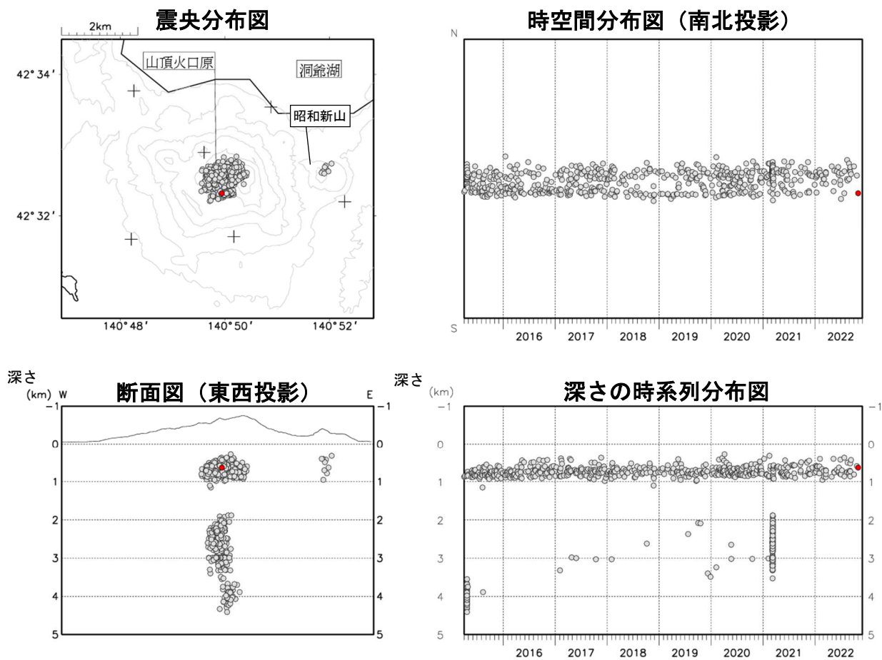
図5 有珠山 火山性地震の震源分布（2015年4月～2022年11月）
