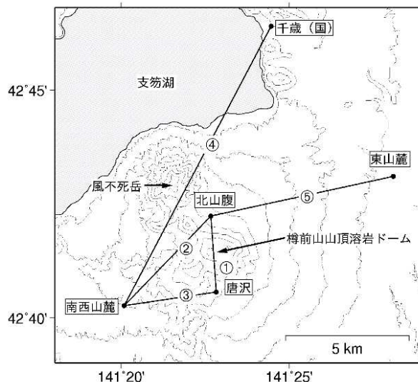
図7 樽前山 GNSS連続観測による基線長変化（2005年1月～2022年9月）及び観測点配置図
