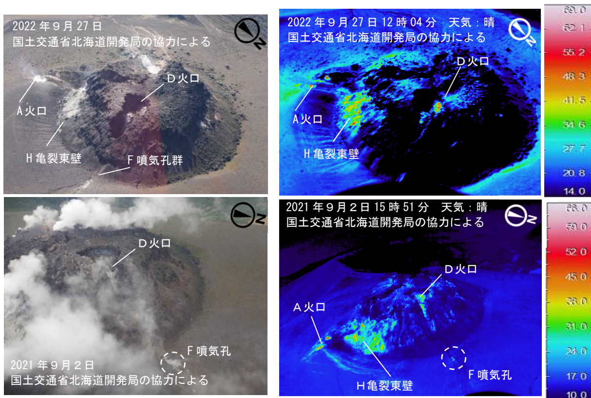
図4 樽前山 赤外熱映像装置による山頂溶岩ドーム東側の地表面温度分布
