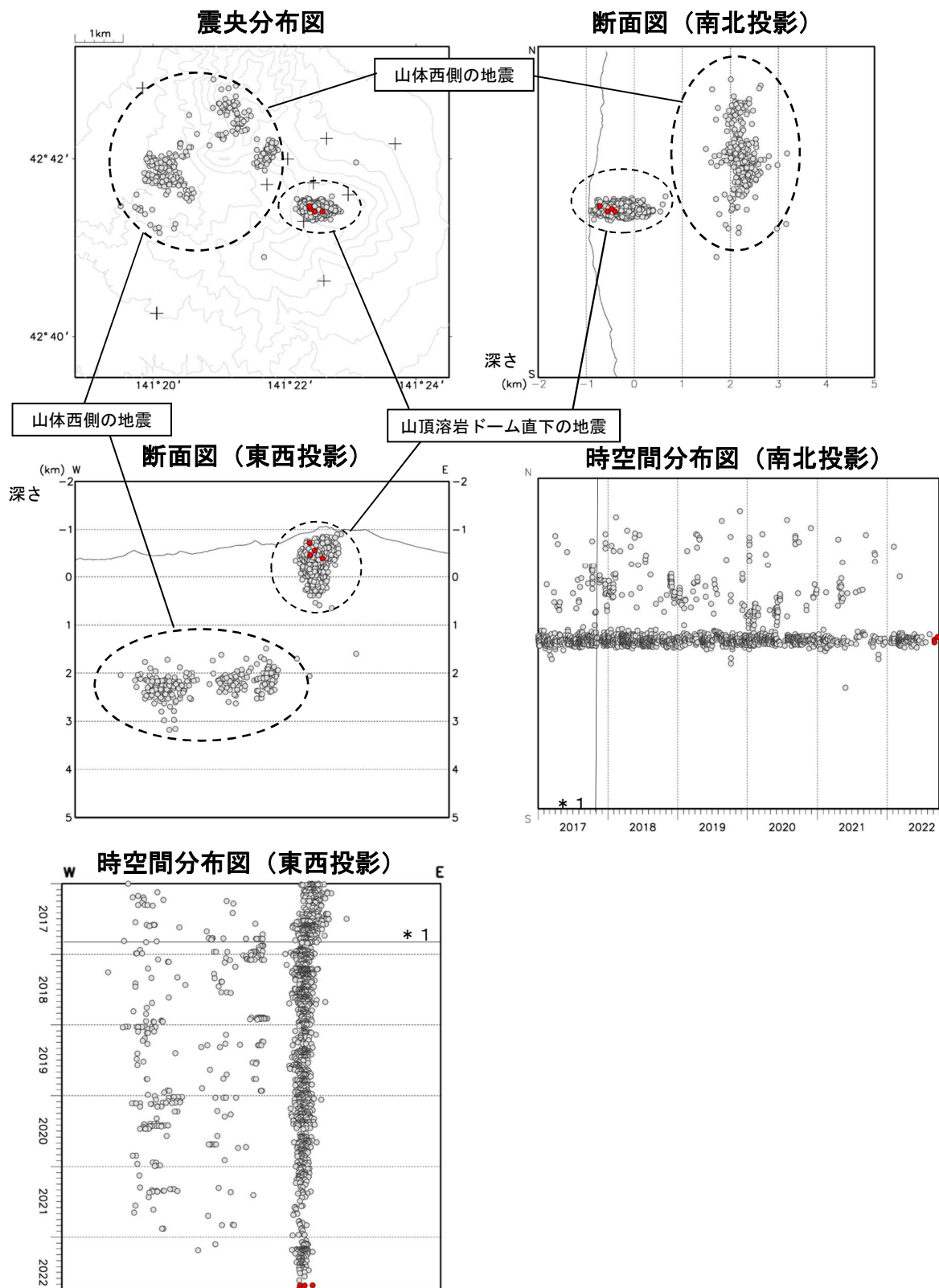
図6 樽前山 火山性地震の震源分布（2017年1月～2022年9月） ○印：2017年1月～2022年8月の震源 ●印：2022年9月の震源 ＋印：地震観測点 2017年10月31日（*1）以降、震源計算に利用する観測点を変更しています。
