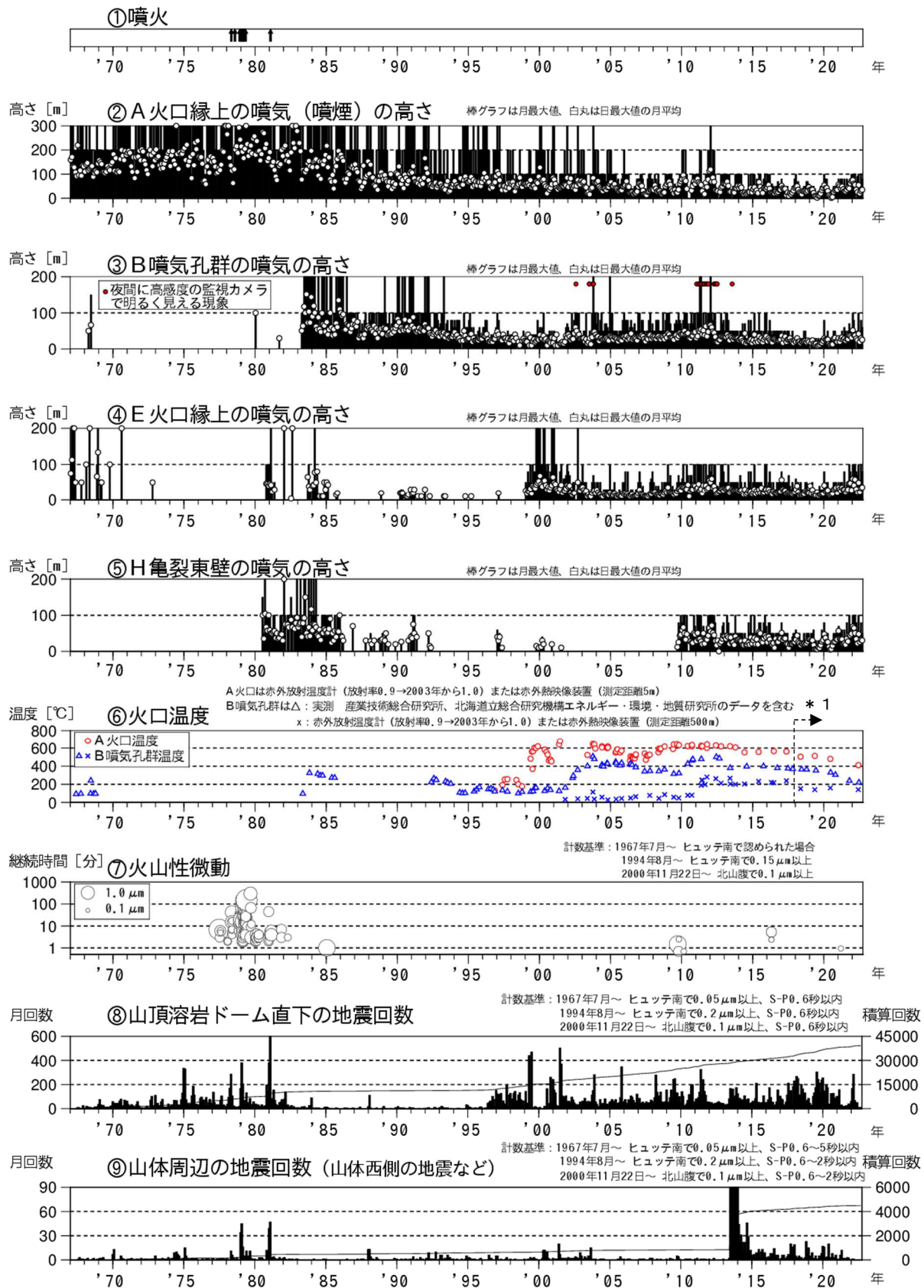
図2 樽前山 火山活動経過図（1967年1月～2022年9月）
