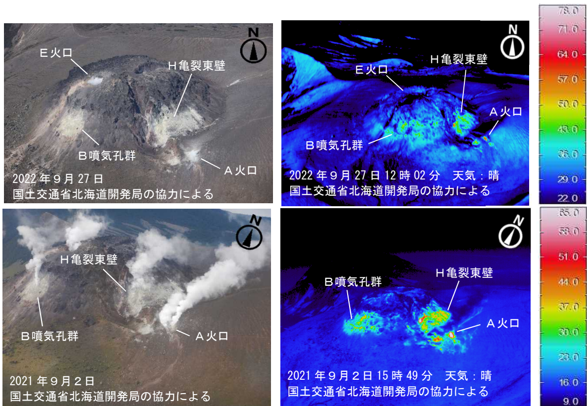
図5 樽前山 赤外熱映像装置による山頂溶岩ドーム南側～南東側の地表面温度分布
