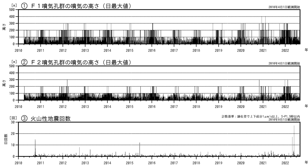
図1 アトサヌプリ 火山活動経過図（2010年4月～2022年8月）
