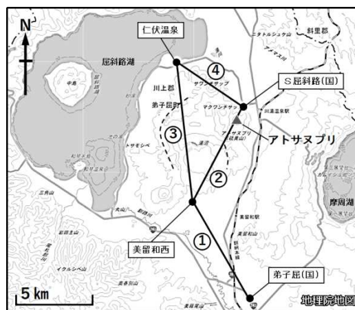
図3 アトサヌプリ GNSS連続観測による基線長変化（2010年10月～2022年8月）及び観測点配置図
