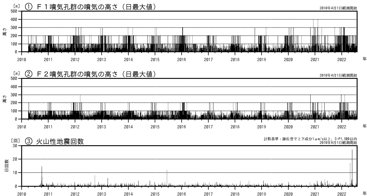
図1 アトサヌプリ 火山活動経過図（2010年4月～2022年7月）
