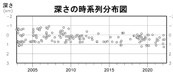
図4 北海道駒ヶ岳 火山性地震の震源分布（2002年12月～2022年6月）
