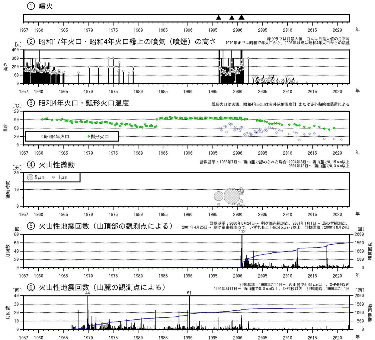
図1 北海道駒ヶ岳 火山活動経過図（1957年1月～2022年6月）
