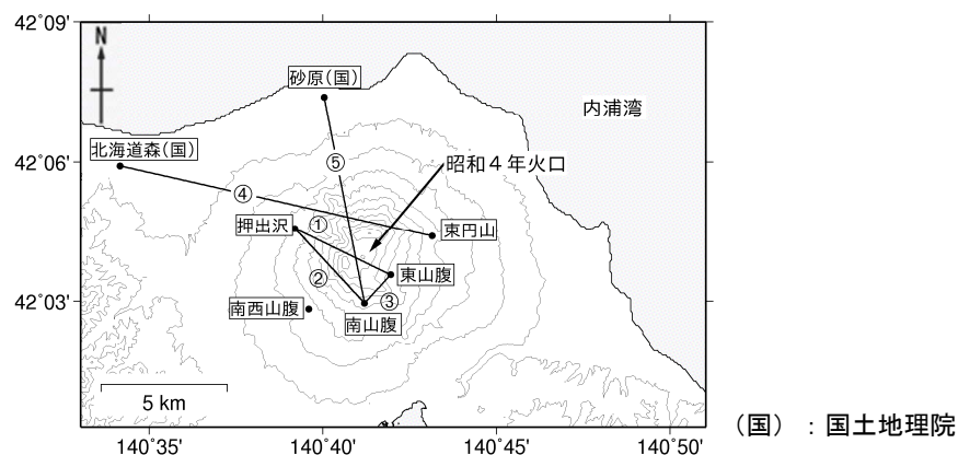
図5 北海道駒ヶ岳 GNSS連続観測による基線長変化（2001年4月～2022年6月）及び観測点配置図 グラフ①～⑤は観測点配置図の基線①～⑤に対応しています。
